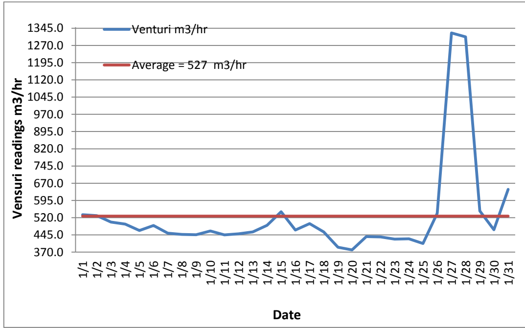
شكل (2) : معدل قراءة عداد فنتشوري (Venture)
