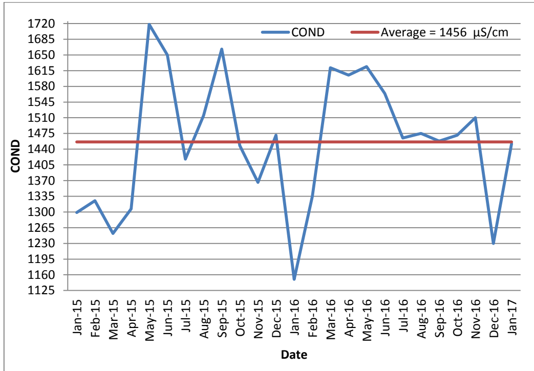
الشكل (15) : معدل قيم الموصلية الكهربائية الشهرية للمياه العادمة الداخلة لمحطة المعالجة
