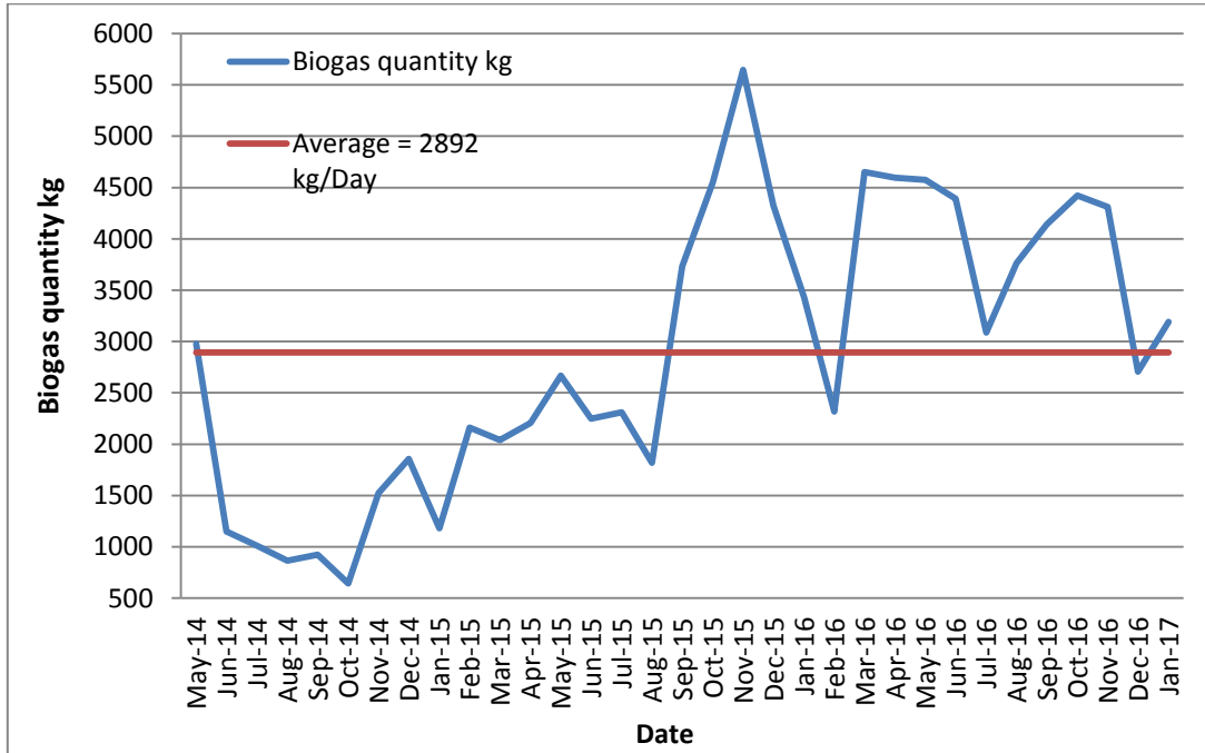
الشكل (11) : متوسط الكميات المنتجة للغاز الحيوي كغم/شهريا
