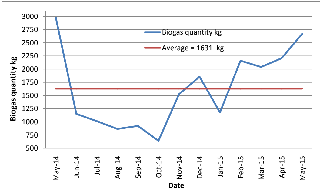
الشكل (11) : متوسط الكميات المنتجة للغاز الحيوي شهرياً Average Monthly Biogas production
