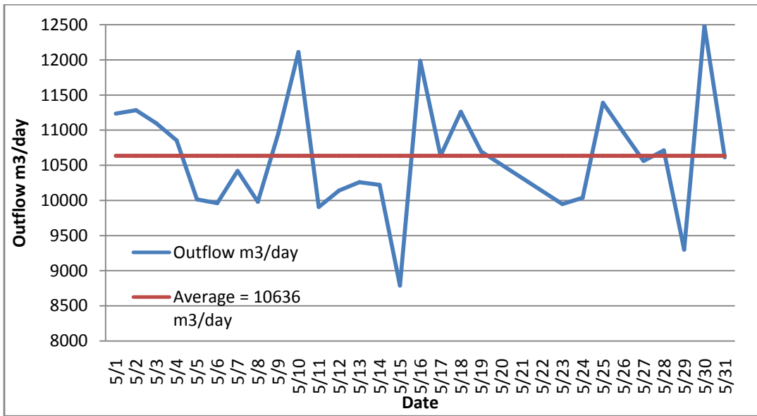
شكل (3) : كمية المياه العادمة الخارجة من المحطة
