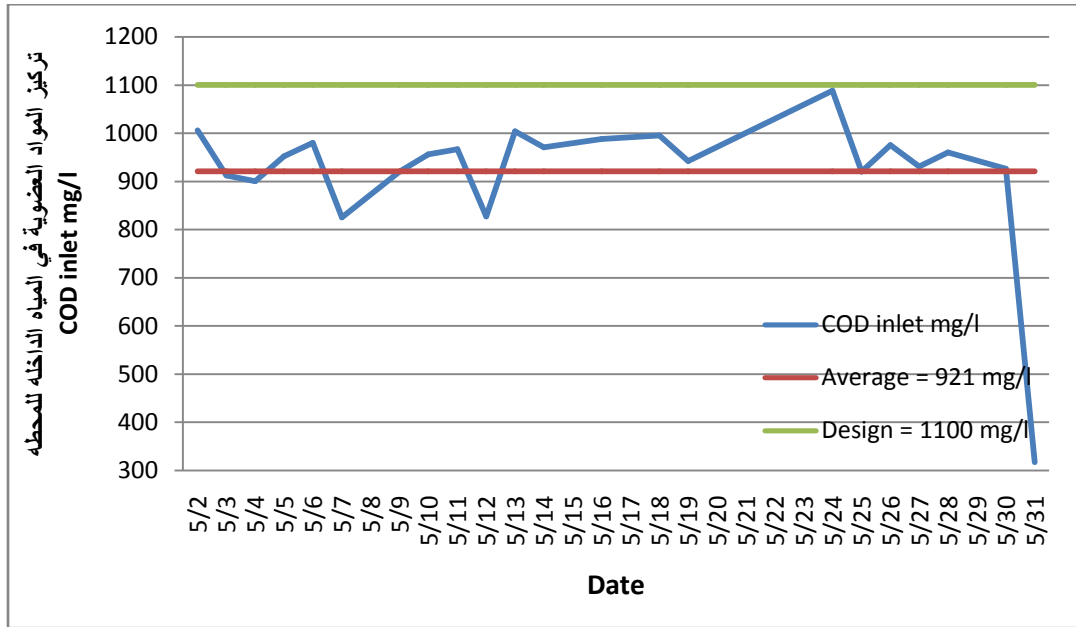
شكل (6) : تركيز المواد العضويه في المياه العادمه الداخله للمحطه
