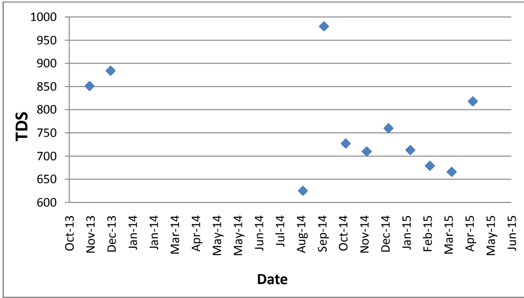
الشكل (16) : بعض القيم الناتجة عن تحليل الأملاح الذائبة للمياه المعالجة
