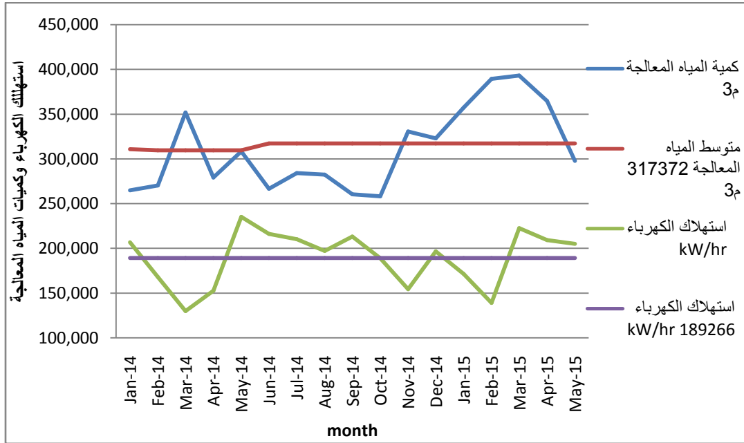
الشكل (14) : معدلي استهلاك الكهرباء والمياه المعالجة
