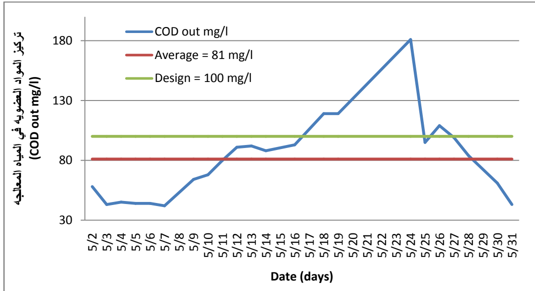
شكل (7) : تركيز المواد العضويه في المياه المعالجه
