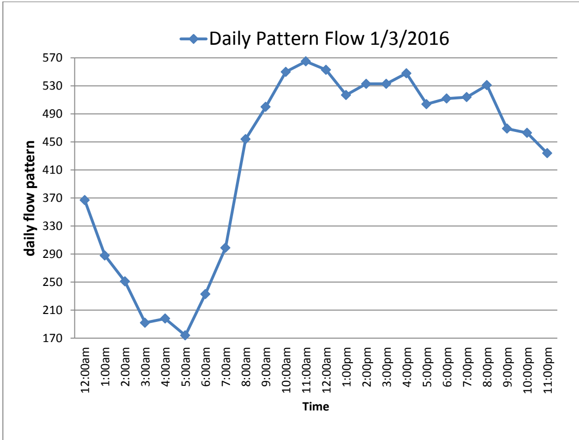
الشكل (1) : كمية المياه العادمة الداخلة خلال 24 ساعة
