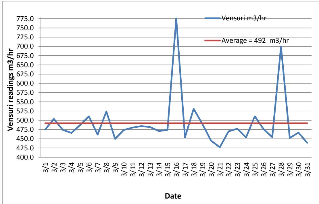
شكل (2) : معدل قراءة عداد فنتشوري (Venture)
