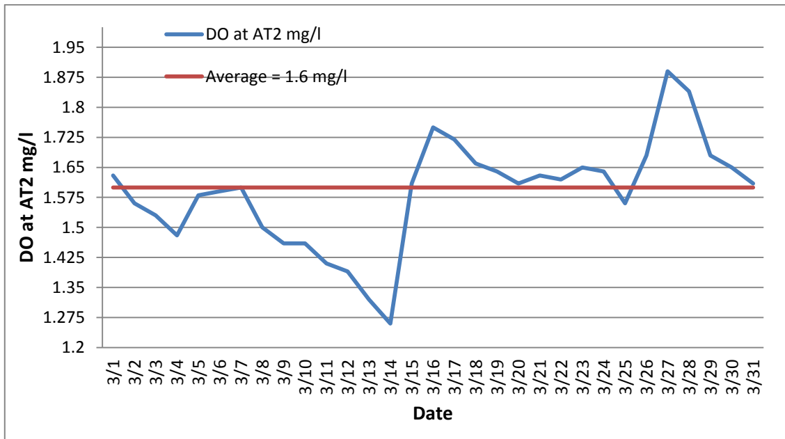
شكل (5) : كمية الأوكسجين المذاب في خزان التهويه 240.2
