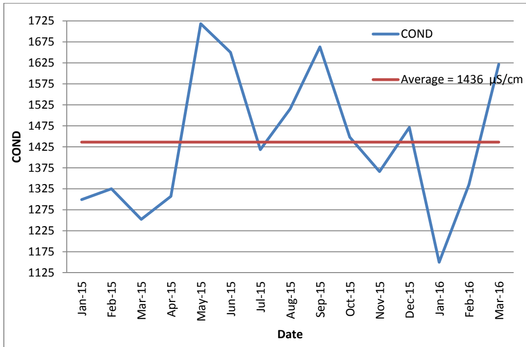
الشكل (15) : معدل قيم التوصيلية الكهربائية الشهرية للمياه العادمة الداخلة لمحطة المعالجة
