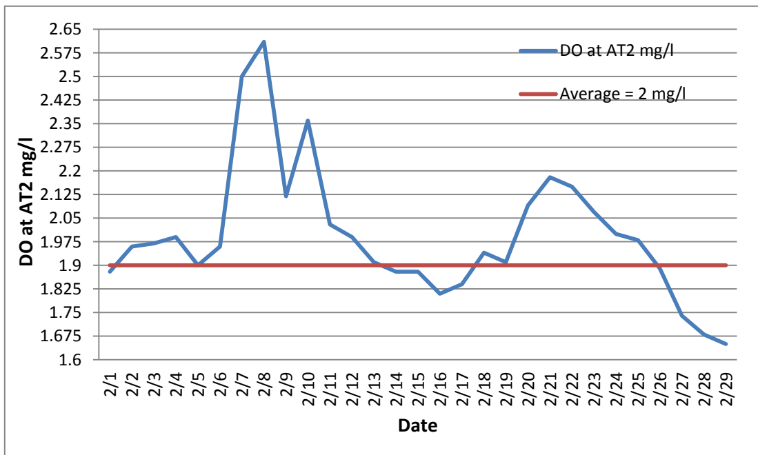
شكل (5) : كمية الأوكسجين المذاب في خزان التهويه 240.2
