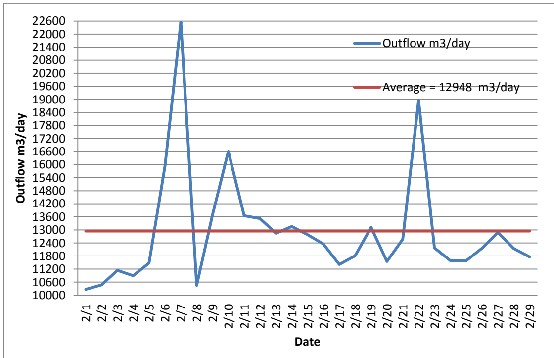
شكل (3) : كمية المياه المعالجة الخارجة من المحطة
