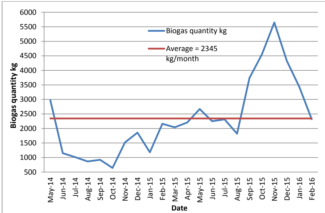
الشكل (11) : متوسط الكميات المنتجة للغاز الحيوي كغم/شهرياً
