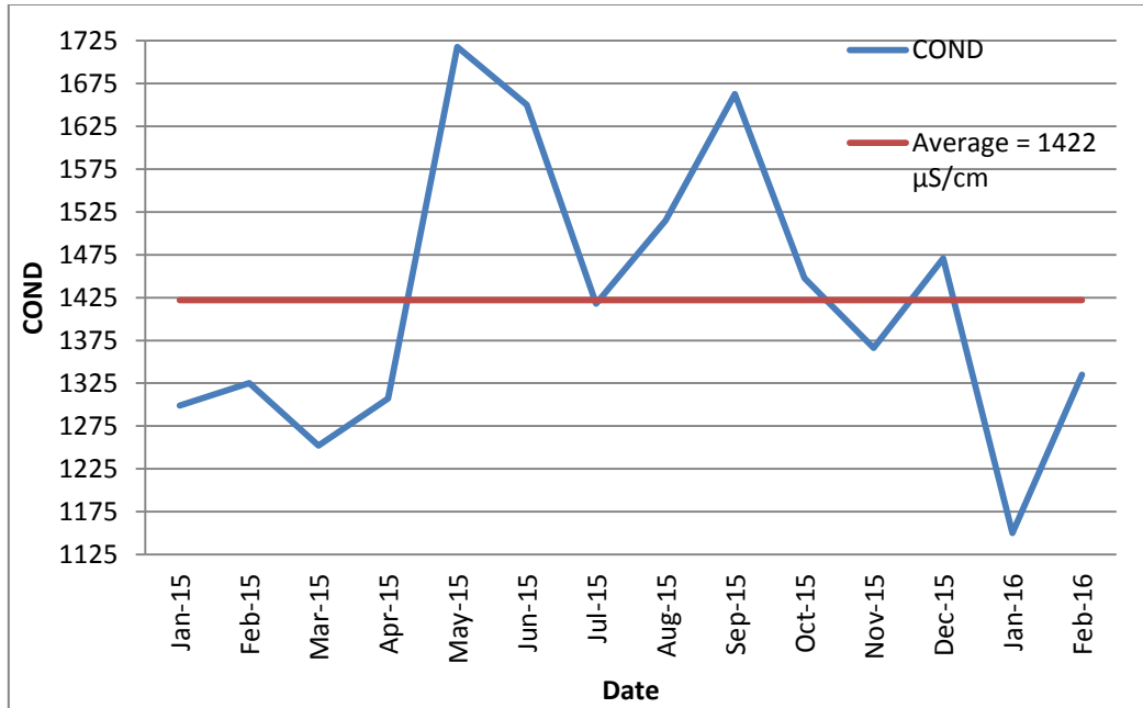
الشكل (15) : معدل قيم الموصلية الكهربائية الشهري للمياه العادمة الداخلة لمحطة المعالجة
