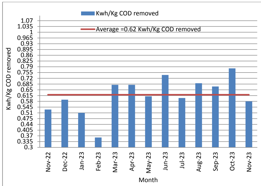
19: يوضح كميات الطاقة الكهربائية المستخدمة بدلالة كيلو واط ساعة لكل كغم COD 2023/11 2022/11
