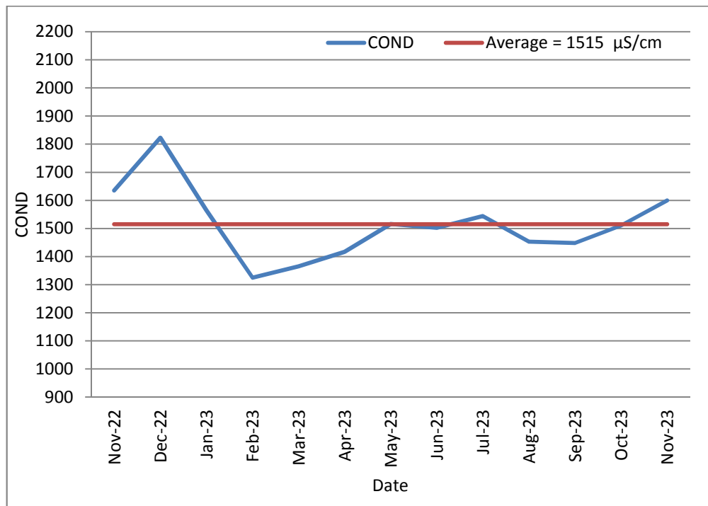
13 : يوضح قيم الموصلية الكهربائية (Conductivity) للمياه العادمة الداخلة 2023/11 2022/11
