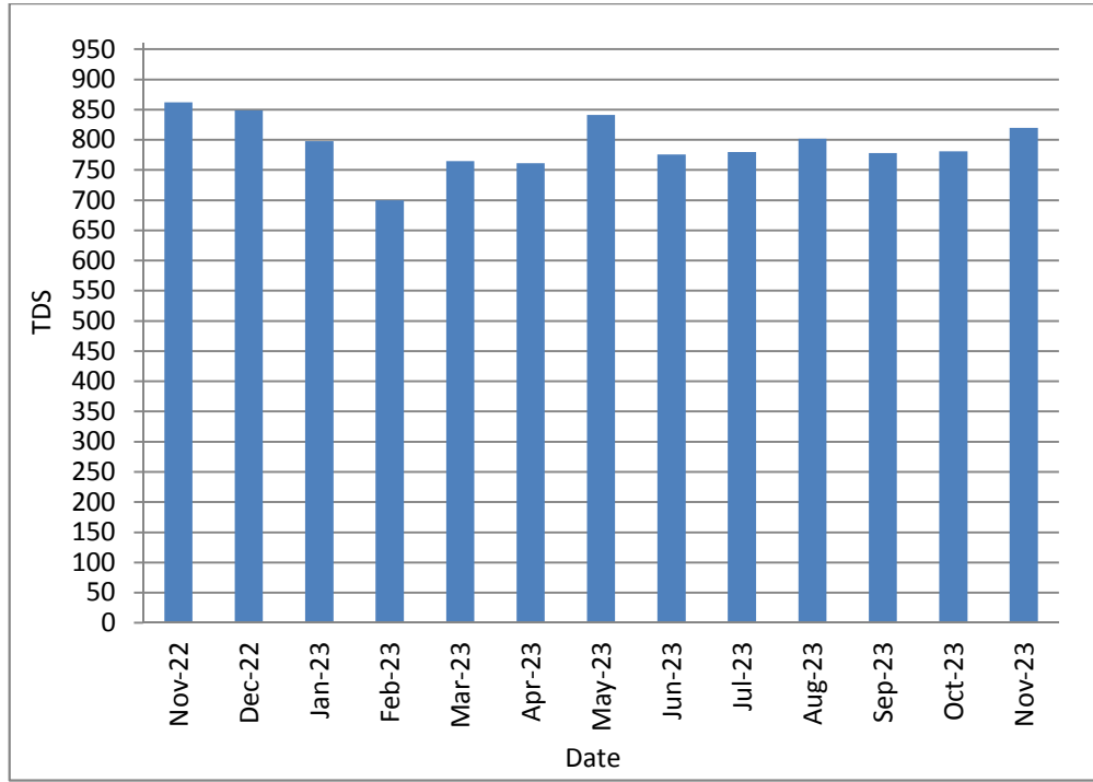
14: يوضح قيم نسبة الاملاح الكلية الذائبة في المياه المعالجة (TDS) 2023/11 2022/11
