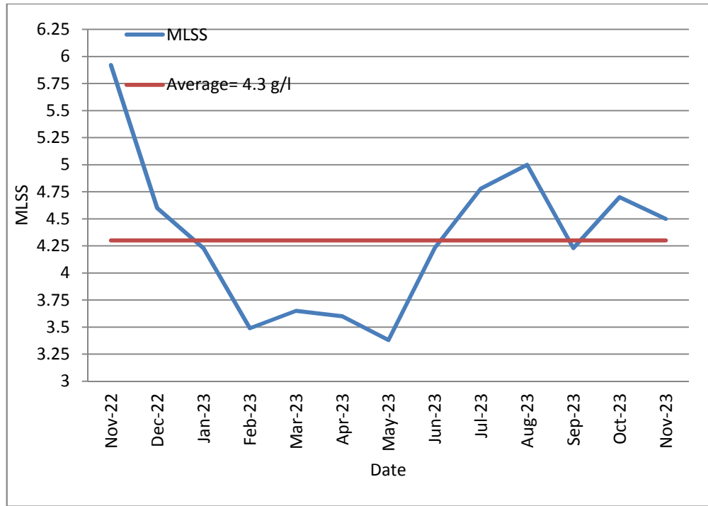
12: يوضح قيم نسبة المواد الصلبة المعلقة الحيوية في خزانات التهوية (MLSS) 2023/11 2022/11
