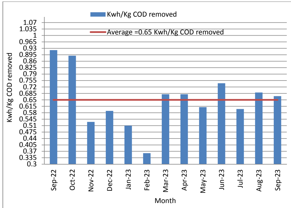
19: يوضح كميات الطاقة الكهربائية المستخدمة بدلالة كيلو واط ساعة لكل كغم COD 2023/9 2022/9
