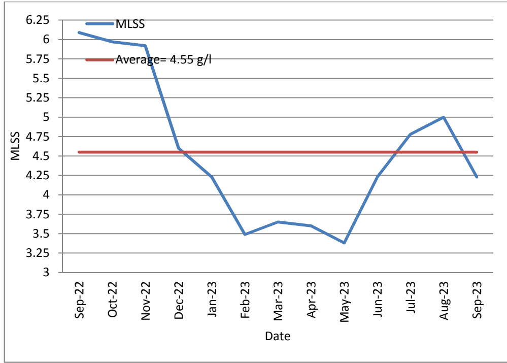
12: يوضح قيم نسبة المواد الصلبة المعلقة الحيوية في خزانات التهوية (MLSS) 2022/9 2023/9
