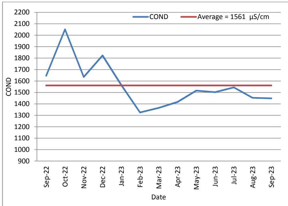
13 : يوضح قيم الموصلية الكهربائية (Conductivity) للمياه العادمة الداخلة 2022/9 2023/9
