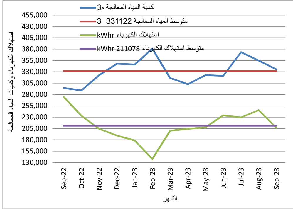
18: يوضح قيمة استهلاك الكهرباء وكمية المياه المعالجة 2023/9 2022/9
