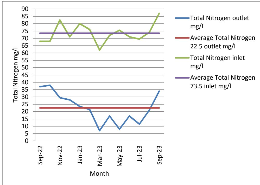
15: يبين فحوصات عملية إزالة النيتروجين 2023/9 2022/9
