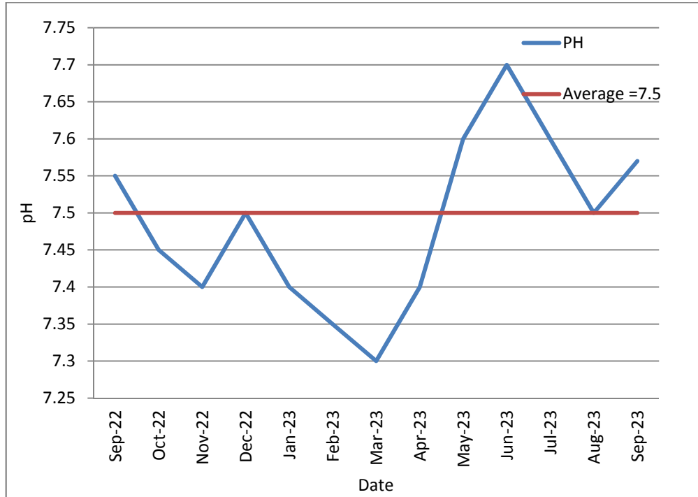
11: بوضوح قيم درجة الحموضة للمياه الداخلة للمحطة (pH) 2023/9 2022/9
