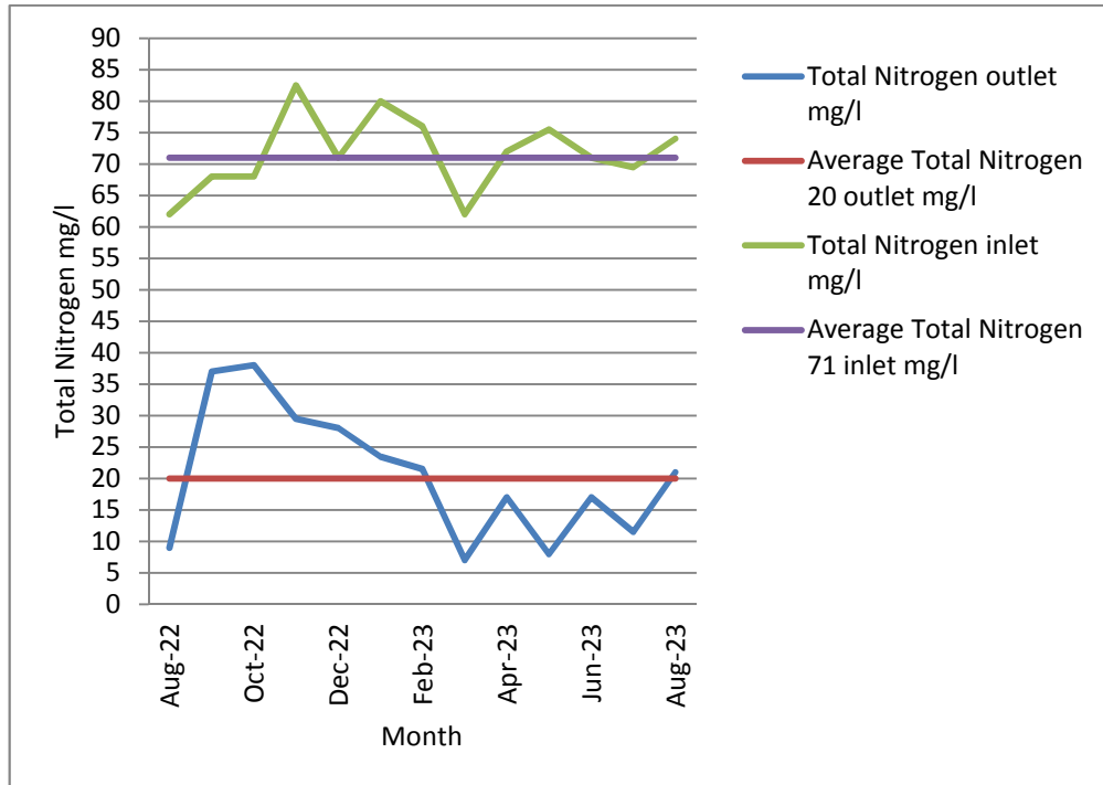
15: يبين فحوصات عملية إزالة النيتروجين 2022/8 2023/8
