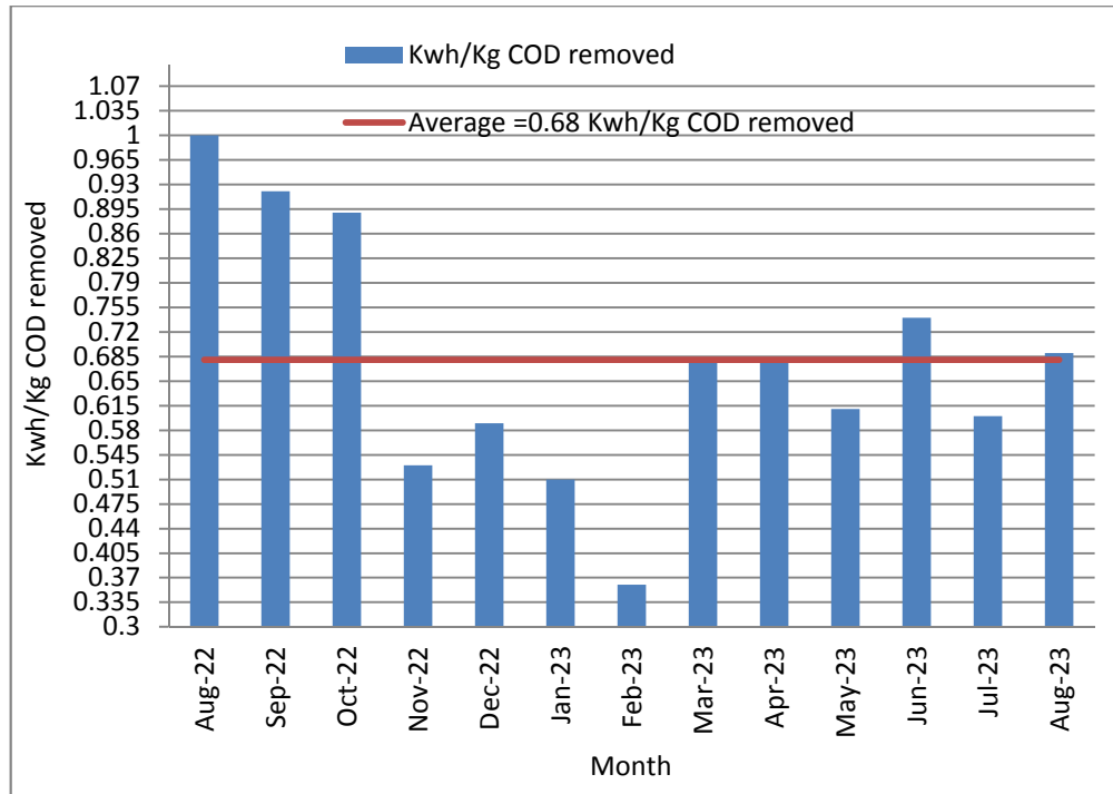
19: يوضح كميات الطاقة الكهربائية المستخدمة بدلالة كيلو واط ساعة لكل كغم COD 2023/8 2022/8
