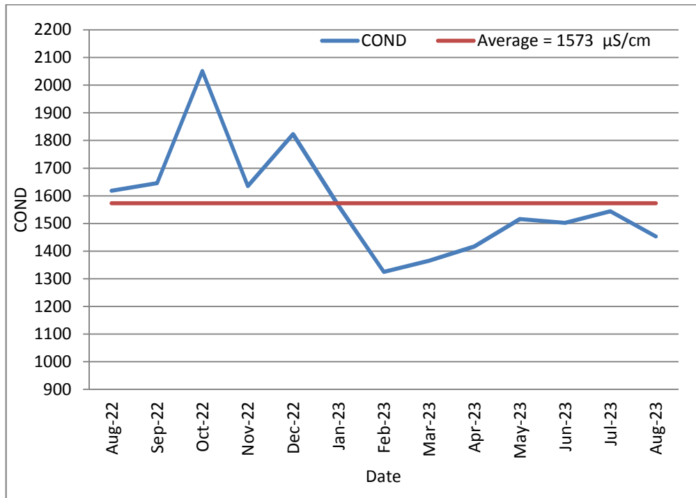
13 : يوضح قيم الموصلية الكهربائية (Conductivity) للمياه العادمة الداخلة 2022/8 2023/8
