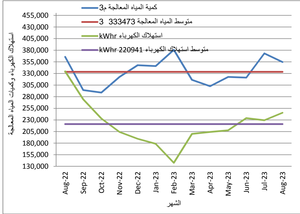
18: يوضح قيمة استهلاك الكهرباء وكمية المياه المعالجة 2023/8 2022/8
