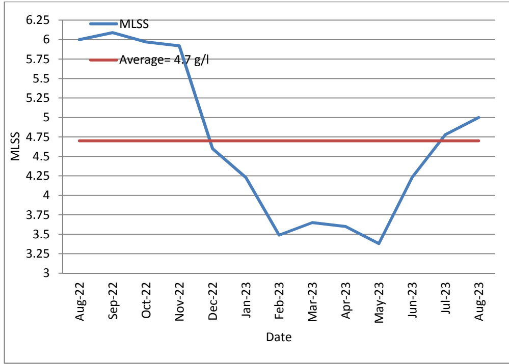
12: يوضح قيم نسبة المواد الصلبة المعلقة الحيوية في خزانات التهوية (MLSS) 2022/8 2023/8
