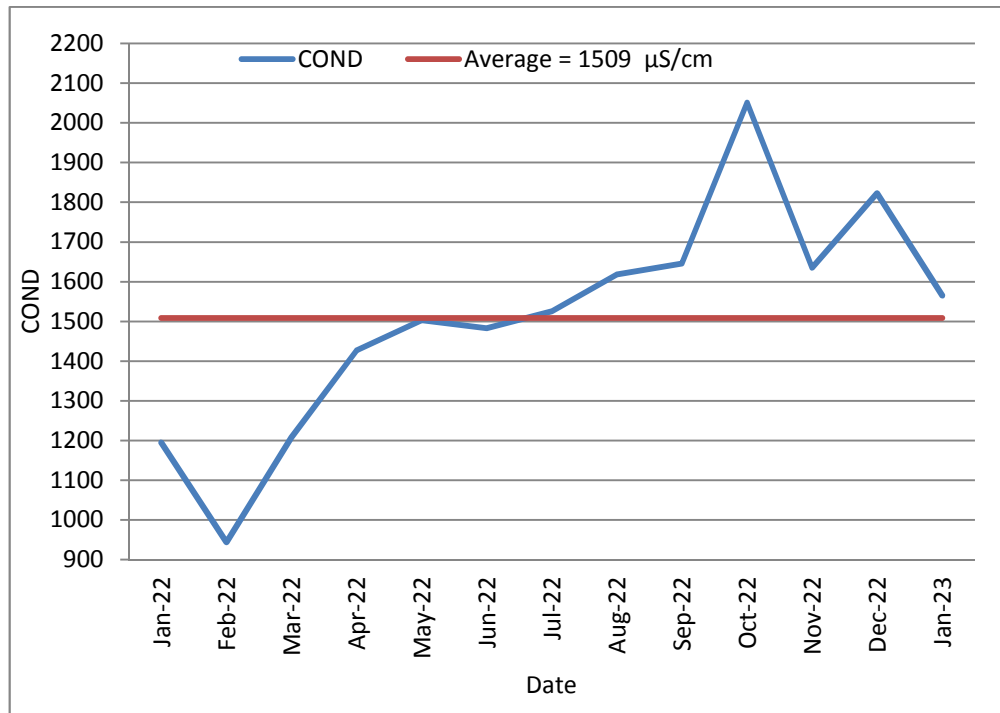
13 : يوضح قيم الموصلية الكهربائية (Conductivity) للمياه العادمة الداخلة 2022/1 2023/1
