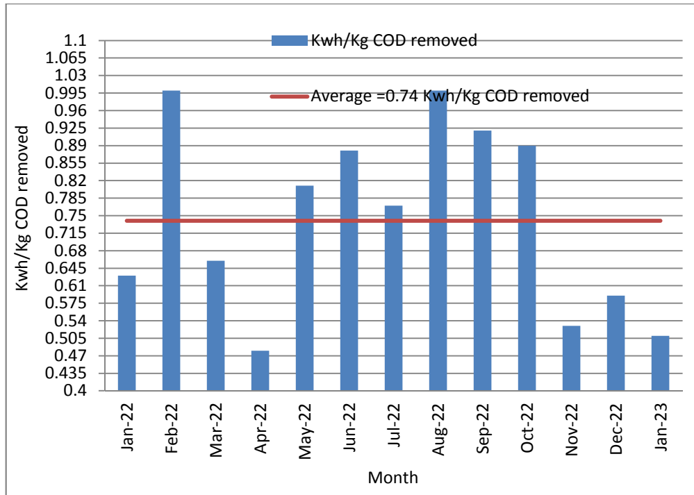
19: يوضح كميات الطاقة الكهربائية المستخدمة بدلالة كيلو واط ساعة لكل كغم COD 2023/1 2022/1
