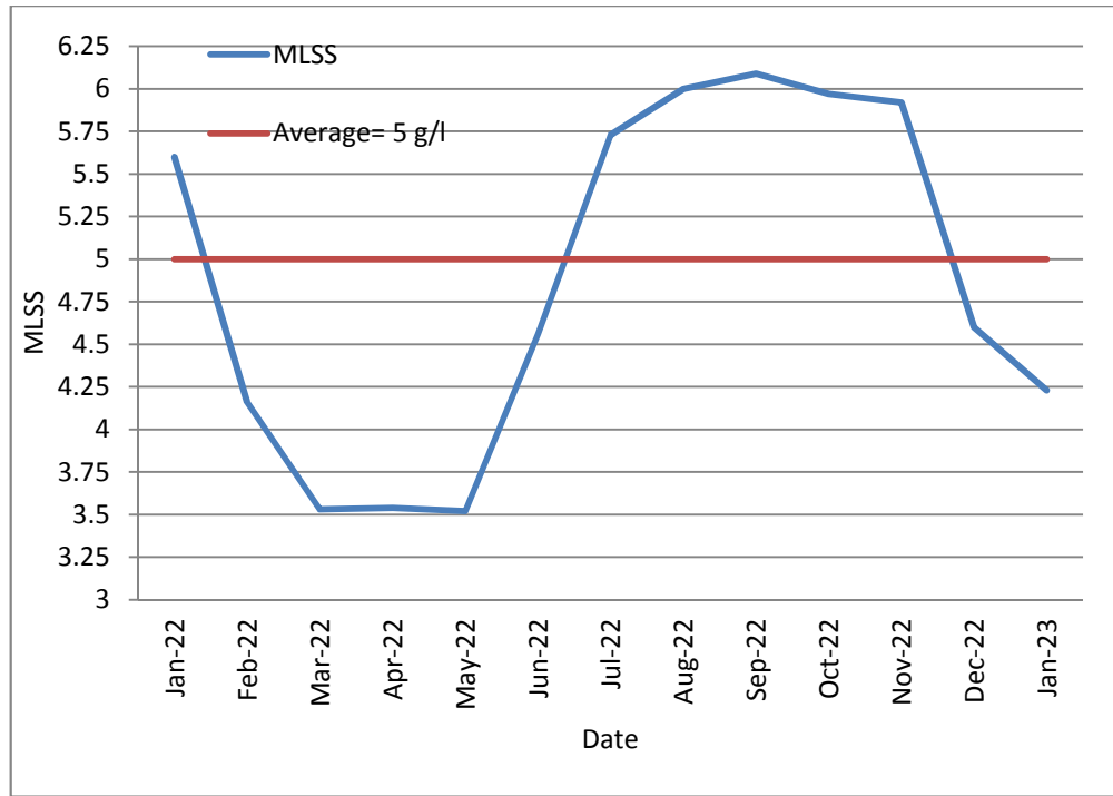
12: يوضح قيم نسبة المواد الصلبة المعلقة الحيوية في خزانات التهوية (MLSS) 2022/1 2023/1
