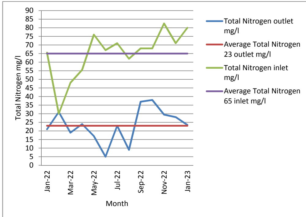
15: يبين فحوصات عملية إزالة النيتروجين 2023/1 2022/1
