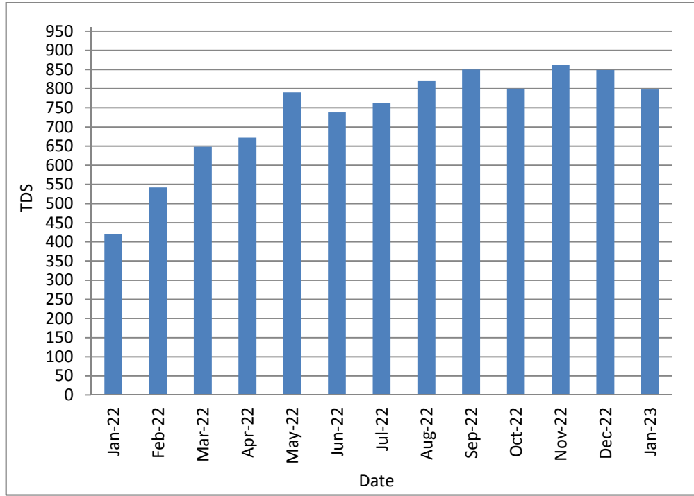
14: يوضح قيم نسبة الاملاح الكلية الذائبة في المياه المعالجة (TDS) 2023/1 2022/1
