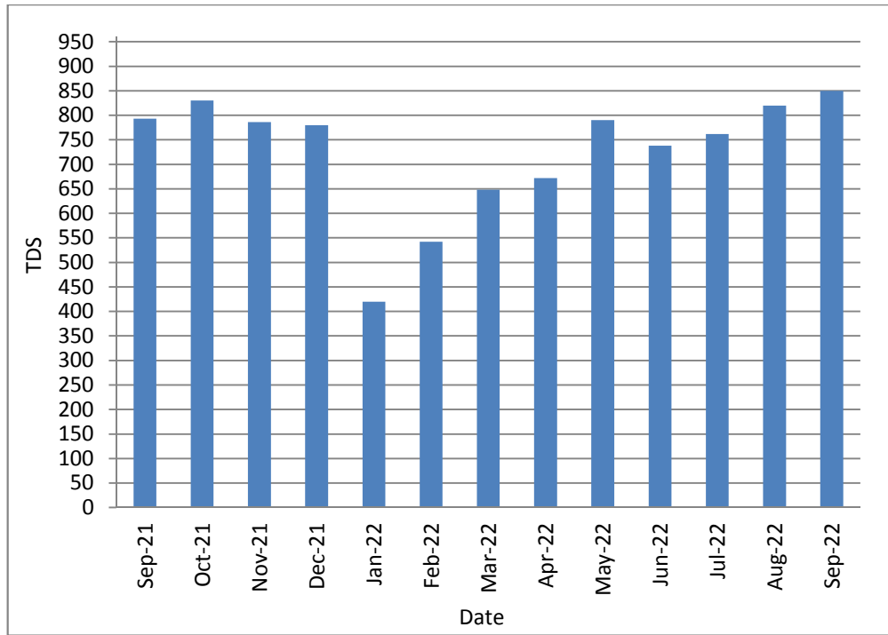
14: يوضح قيم نسبة الاملاح الكلية الذائبة في المياه المعالجة (TDS) 2022/9 2021/9
