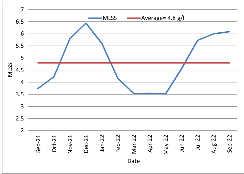
12: يوضح قيم نسبة المواد الصلبة المعلقة الحيوية في خزانات التهوية (MLSS) 2022/9 2021/9
