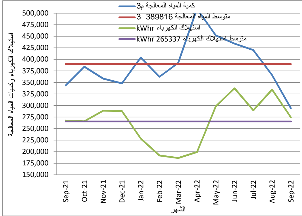
18: يوضح قيمة استهلاك الكهرباء وكمية المياه المعالجة 2022/9 2021/9
