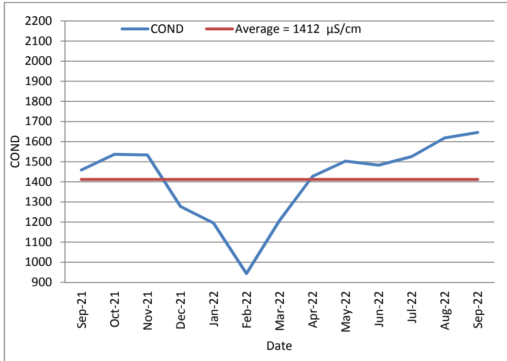
13 : يوضح قيم الموصلية الكهربائية (Conductivity) للمياه العادمة الداخلة 2022/9 2021/9
