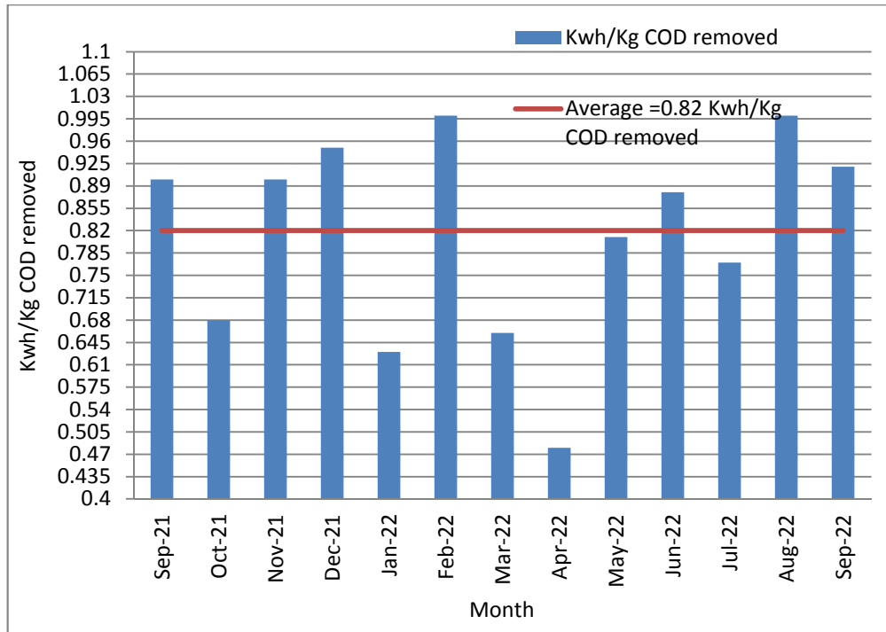
19: يوضح كميات الطاقة الكهربائية المستخدمة بدلالة كيلو واط ساعة لكل كغم COD 2022/9 2021/9
