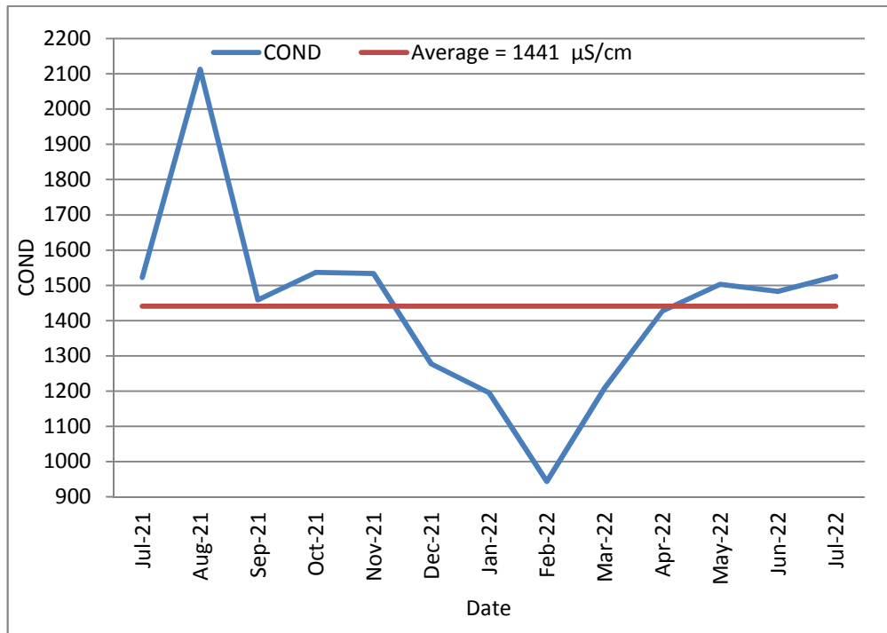
13 : يوضح قيم الموصلية الكهربائية (Conductivity) للمياه العادمة الداخلة 2021/7 2022/7
