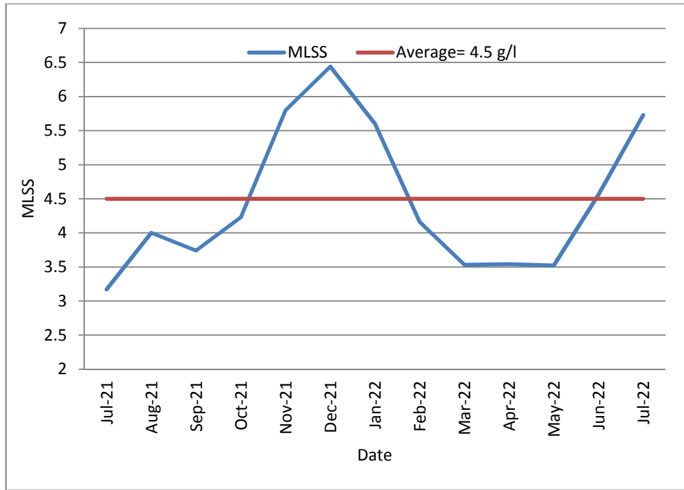
12: يوضح قيم نسبة المواد الصلبة المعلقة الحيوية في خزانات التهوية ( MLSS) 2021/7 2022/7
