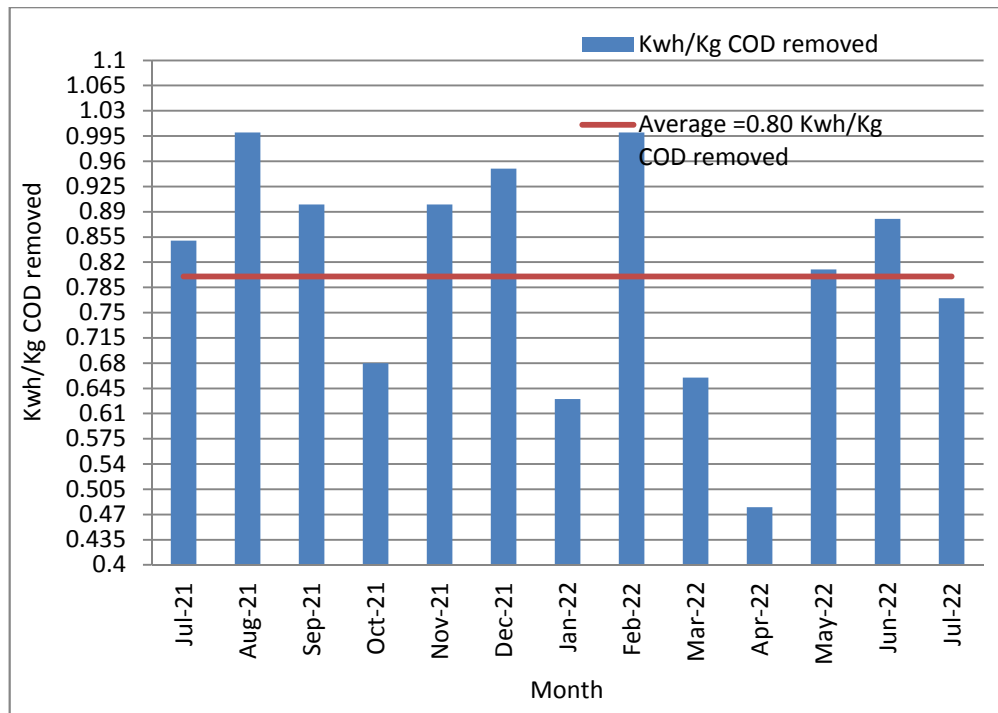
19: يوضح كميات الطاقة الكهربائية المستخدمة بدلالة كيلو واط ساعة لكل كغم COD 2022/7 2021/7
