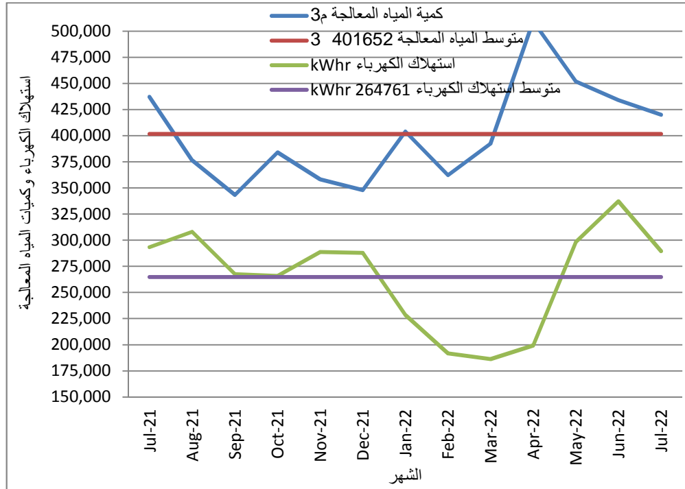
18: يوضح قيمة استهلاك الكهرباء وكمية المياه المعالجة 2022/7 2021/7
