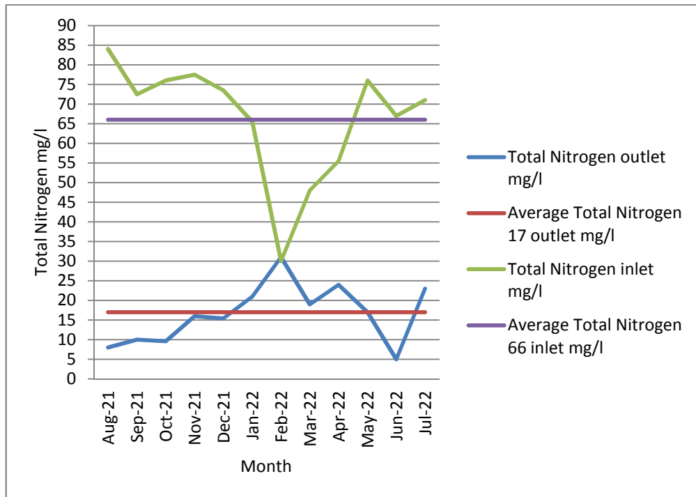
15: يبين فحوصات عملية إزالة النيتروجين 2022/7 2021/7
