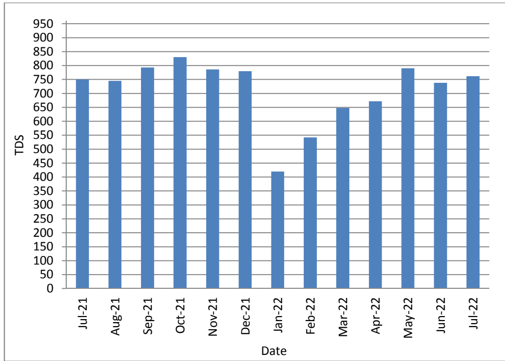
14: يوضح قيم نسبة الاملاح الكلية الذائبة في المياه المعالجة (TDS) 2022/7 2021/7
