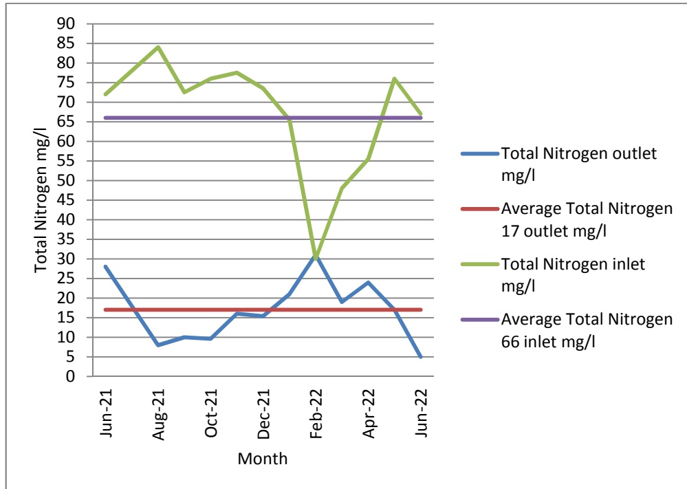
15: يبين فحوصات عملية إزالة النيتروجين 2022/6 2021/6
