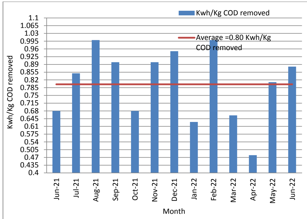
19: يوضح كميات الطاقة الكهربائية المستخدمة بدلالة كيلو واط ساعة لكل كغم COD 2022/6 2021/6
