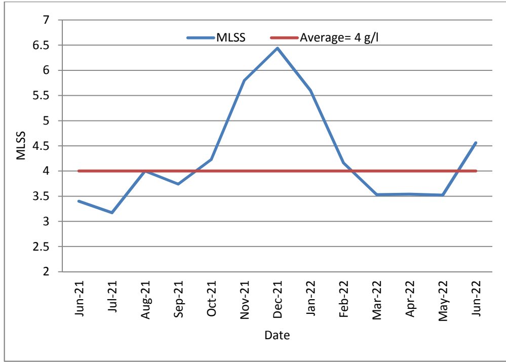
12: يوضح قيم نسبة المواد الصلبة المعلقة الحيوية في خزانات التهوية (MLSS) 2021/6 2022/6
