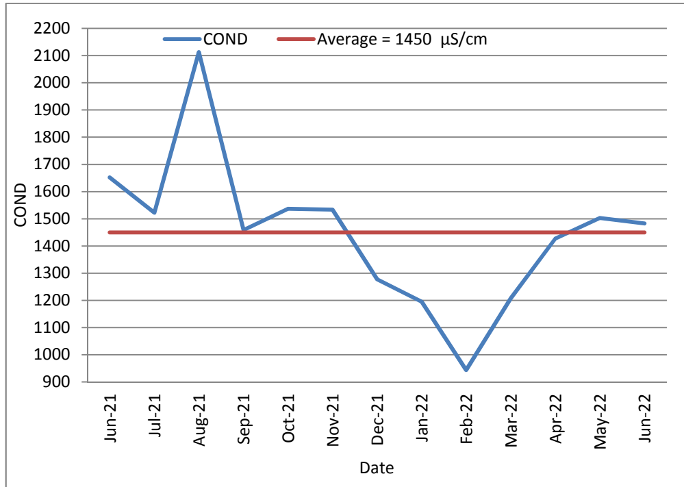
13 : يوضح قيم الموصلية الكهربائية (Conductivity) للمياه العادمة الداخلة 2021/6 2022/6
