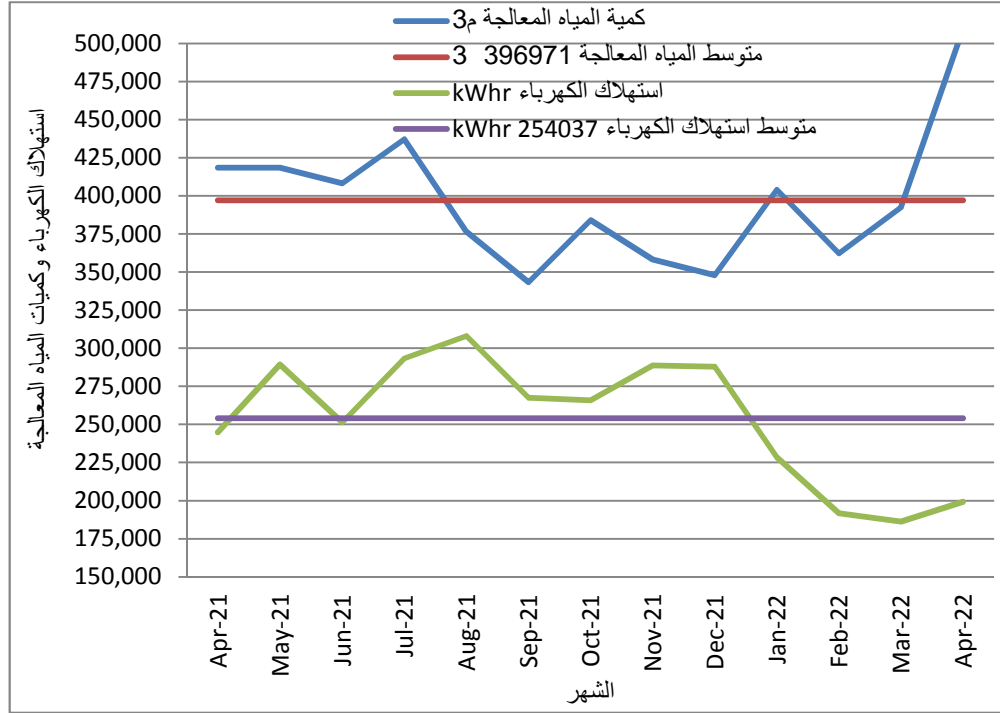
18: يوضح قيمة استهلاك الكهرباء وكمية المياه المعالجة 2022/4 2021/4
