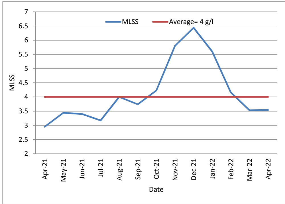
12: يوضح قيم نسبة المواد الصلبة المعلقة الحيوية في خزانات التهوية (MLSS) 2021/4 2022/4
