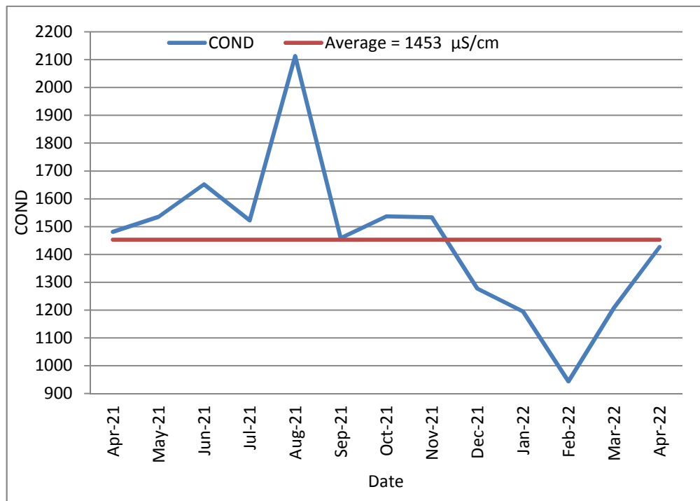
13 : يوضح قيم الموصلية الكهربائية (Conductivity) للمياه العادمة الداخلة 2021/4 2022/4
