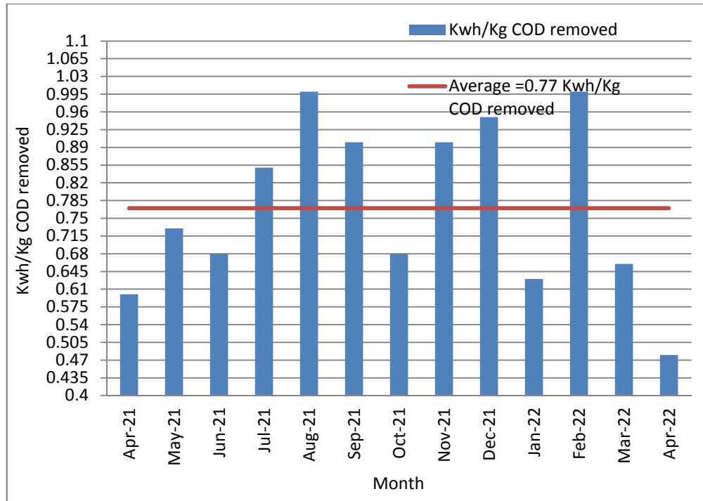
19: يوضح كميات الطاقة الكهربائية المستخدمة بدلالة كيلو واط ساعة لكل كغم COD 2022/4 2021/4
