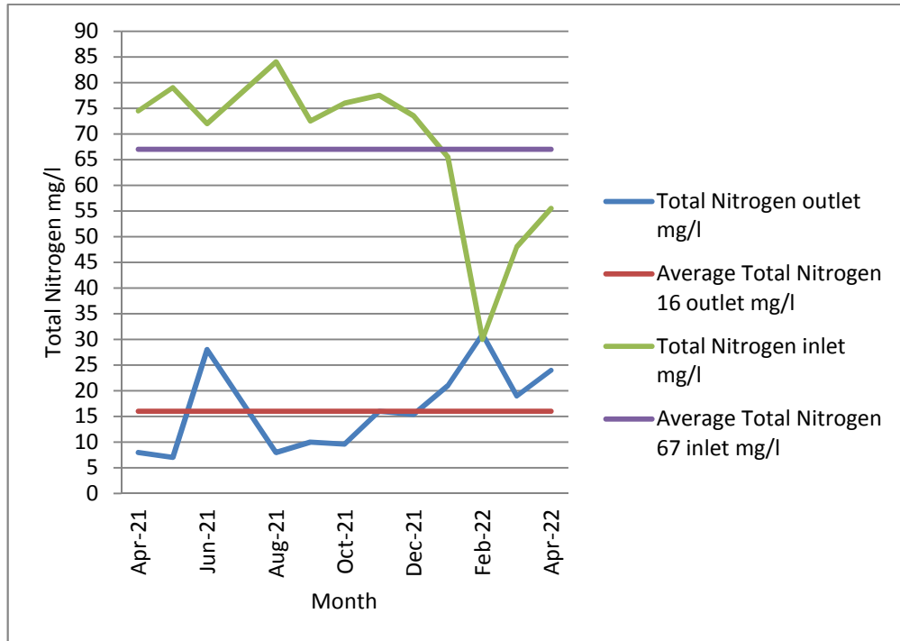
15: يبين فحوصات عملية إزالة النيتروجين 2022/4 2021/4
