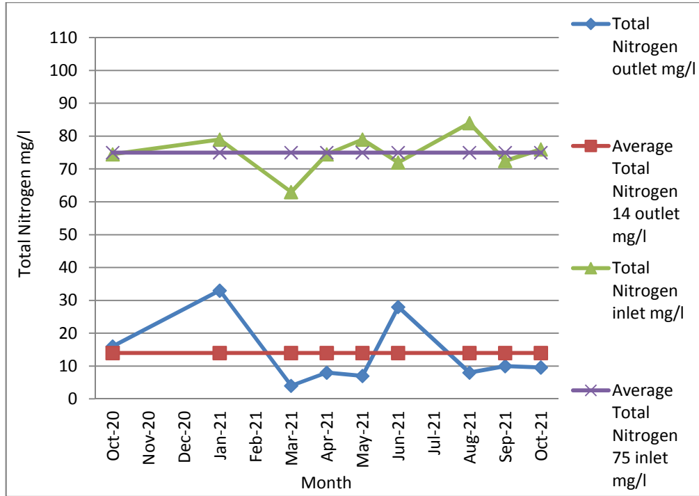
15: يبين فحوصات عملية إزالة النيتروجين 2020/10 2021/10 مع العلم بانه لم يتم عمل فحوصات لبعض الشهور نظرا لـ ( )
