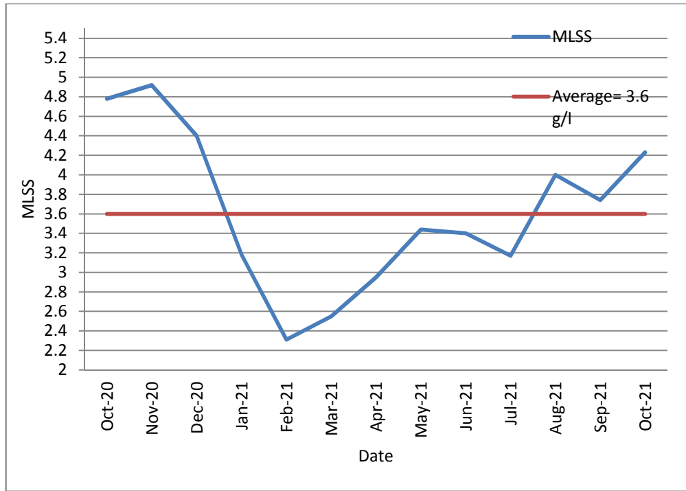
12: يوضح قيم نسبة المواد الصلبة المعلقة الحيوية في خزانات التهوية (MLSS) 2020/10 2021/10
