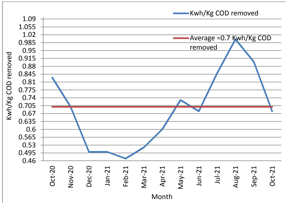
19: يوضح كميات الطاقة الكهربائية المستخدمة بدلالة كيلو واط ساعة لكل كغم COD 2021/10 2020/10
