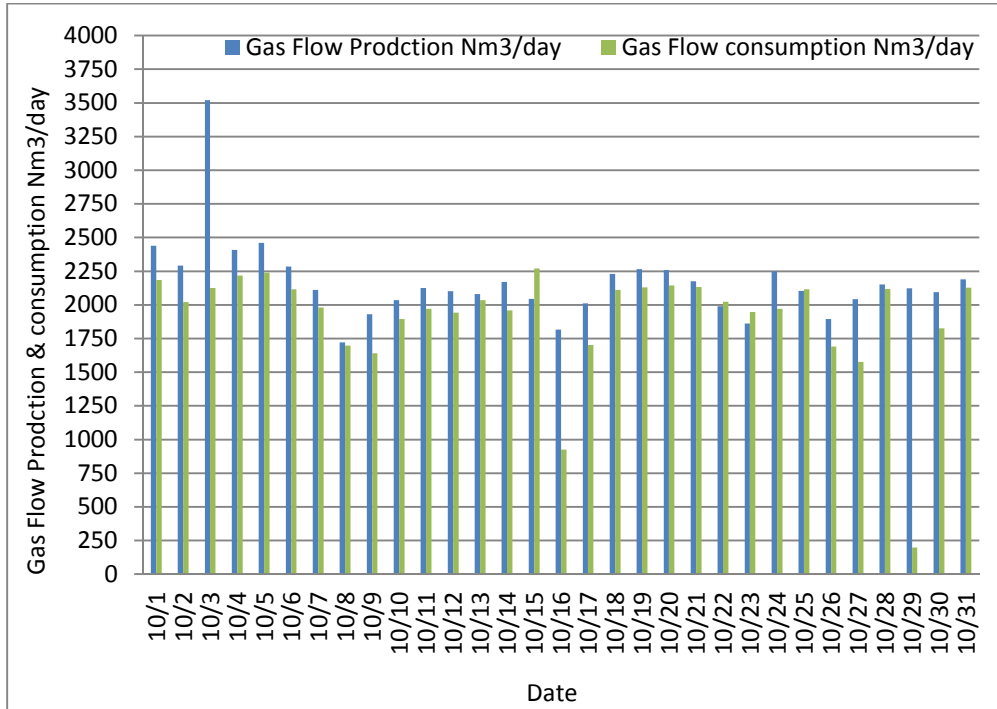
17: بوضوح كمية الغاز الناتج والكمية المستهلكة CHP لشهر تشرين اول والفرق بينهما والذي يتم استخدامه للبويلر درجة حرارة الهاضم اللاهوائي
