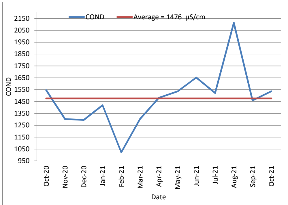
13 : يوضح قيم الموصلية الكهربائية (Conductivity) للمياه العادمة الداخلة 2020/10 2021/10
