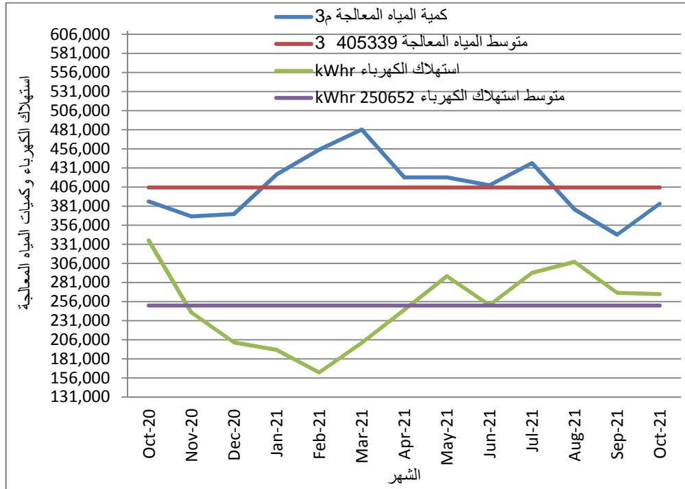
18: يوضح قيمة استهلاك الكهرباء وكمية المياه المعالجة 2021/10 2020/10
