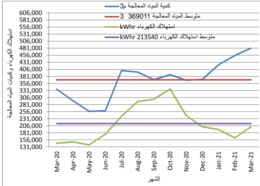
18: يوضح قيمة استهلاك الكهرباء وكمية المياه المعالجة 2021/3 2020/3
