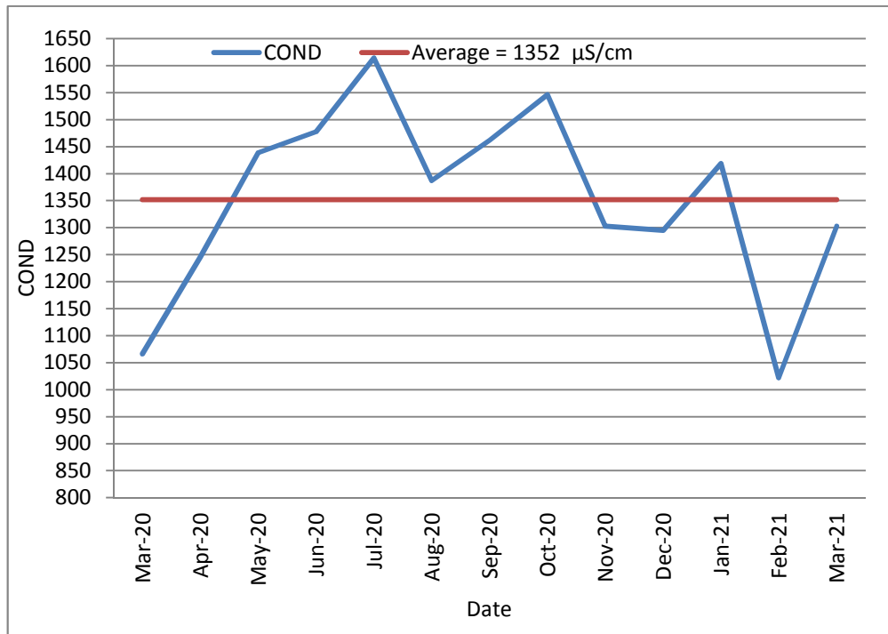
13 : يوضح قيم الموصلية الكهربائية (Conductivity) للمياه العادمة 2020/3 2021/3
