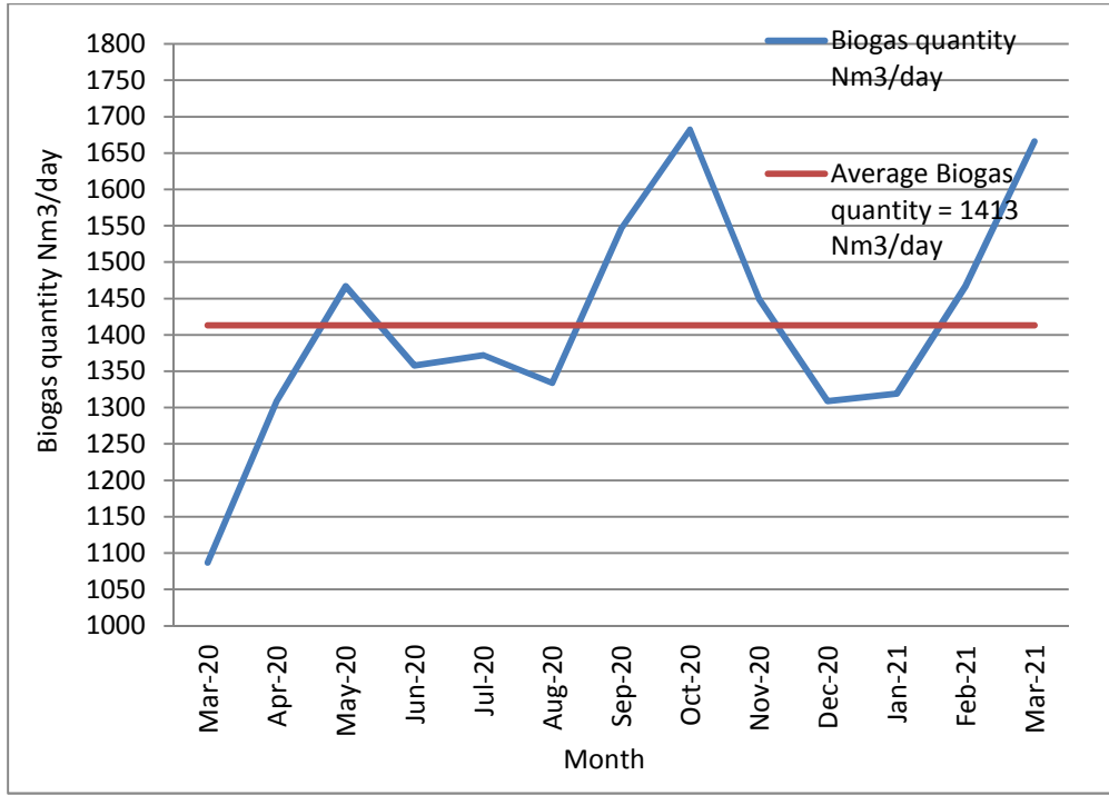
16: يوضح الكميات المنتجة من الغاز الحيوي يومياً 2020/3 2021/3
