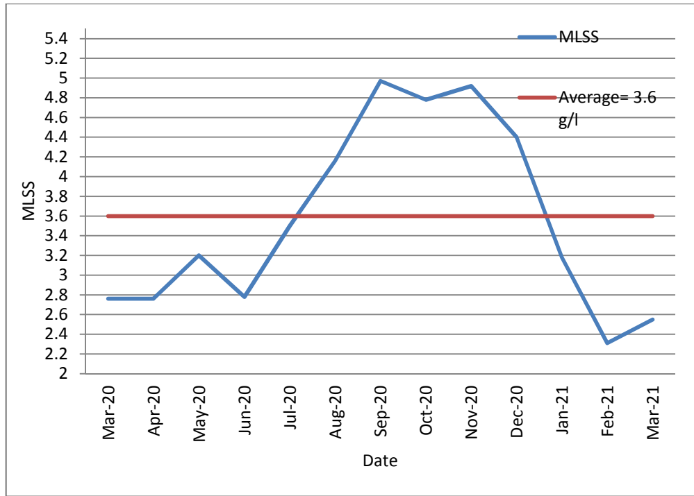
12: يوضح قيم نسبة المواد الصلبة المعلقة الحيوية في خزانات التهوية (MLSS) 2020/3 2021/3
