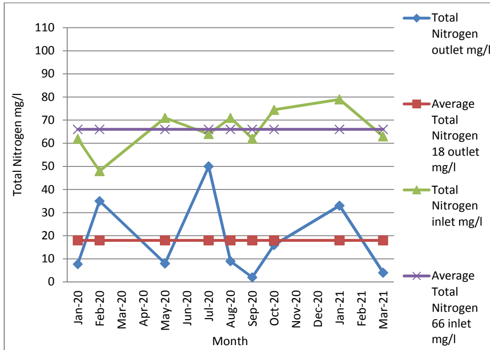
15: يبين فحوصات عملية إزالة النيتروجين 2020/3 2021/3 مع العلم بانه في شهور 3 4 6 11 12 2020/ وشهر 2021/2 لم يتم ( - )
