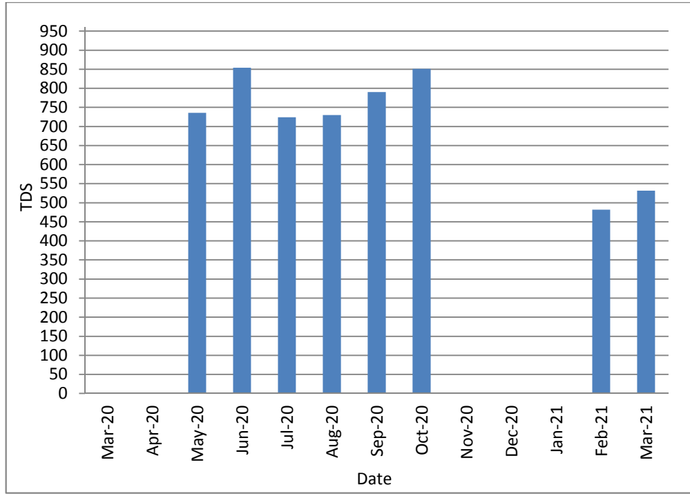
14: يوضح قيم نسبة الاملاح الكلية الذائبة في المياه المعالجة (TDS) 2020/3 2021/3 العلم بانه في شهور 3 4 11 2020/ 12 وشهر 2021/1 لم يتم عمل فحص ( - )
