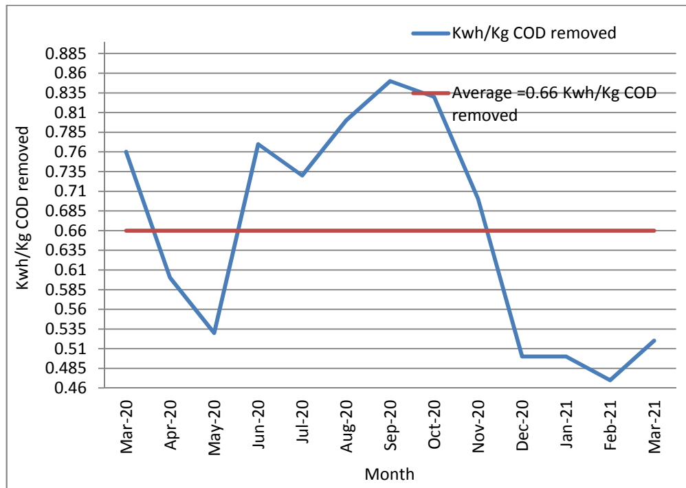
19: يوضح كميات الطاقة الكهربائية المستخدمة بدلالة كيلو واط ساعة لكل كغم COD 2021/3 2020/3
