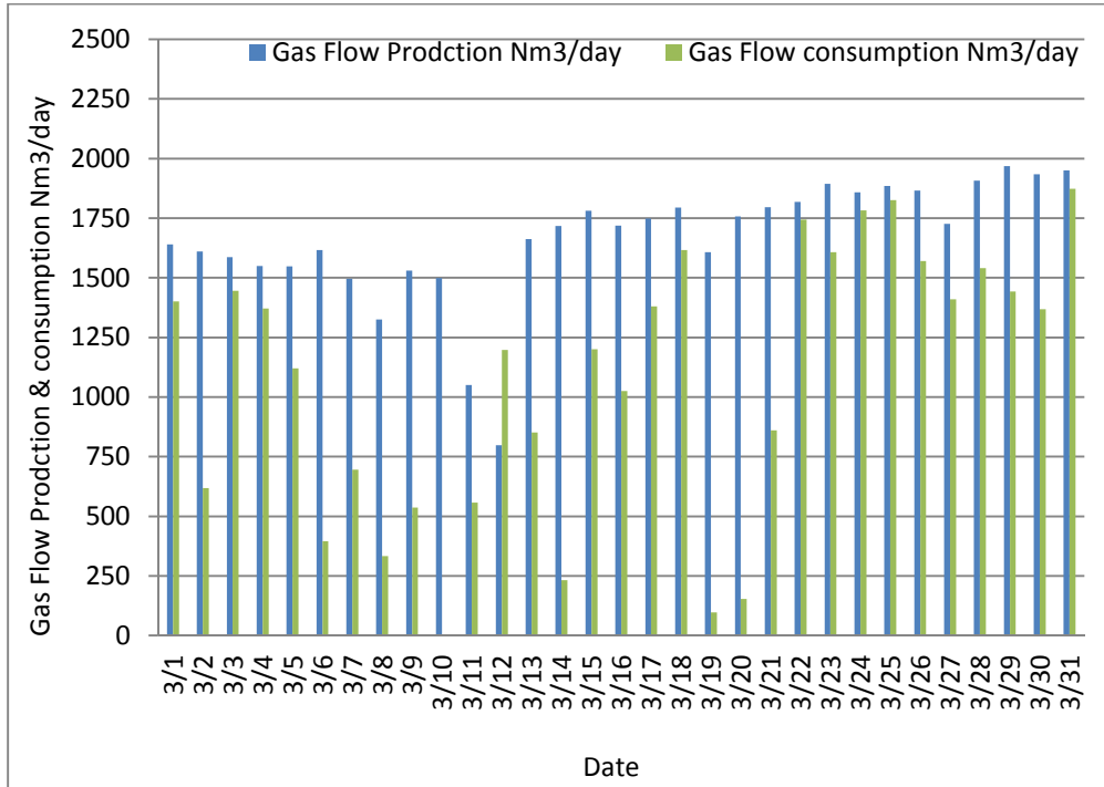
17: يوضح كمية الغاز الناتج والكمية المستهلكة CHP لشهر والفرق بينهما والذي يتم استخدامه للبويلر درجة حرارة الهاضم اللاهوائي
