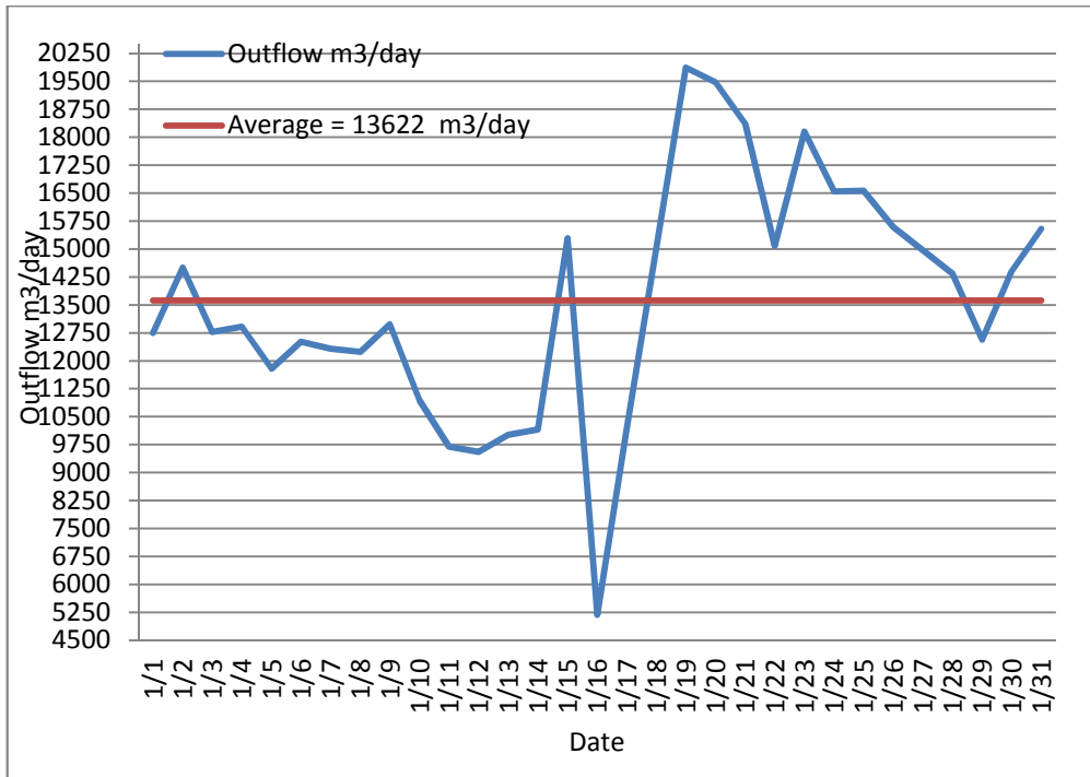
3 : يبين كمية المياه يوميا من المحط .
