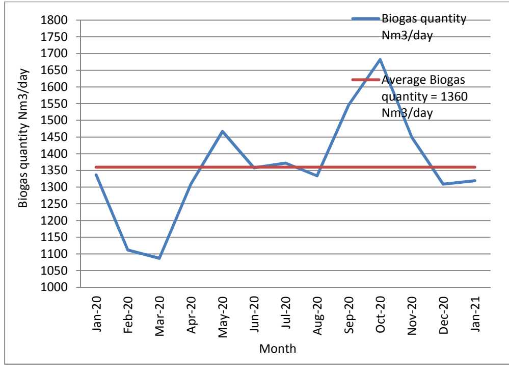
16: يوضح الكميات المنتجة من الغاز الحيوي يوميا 2020/1 2021/1
