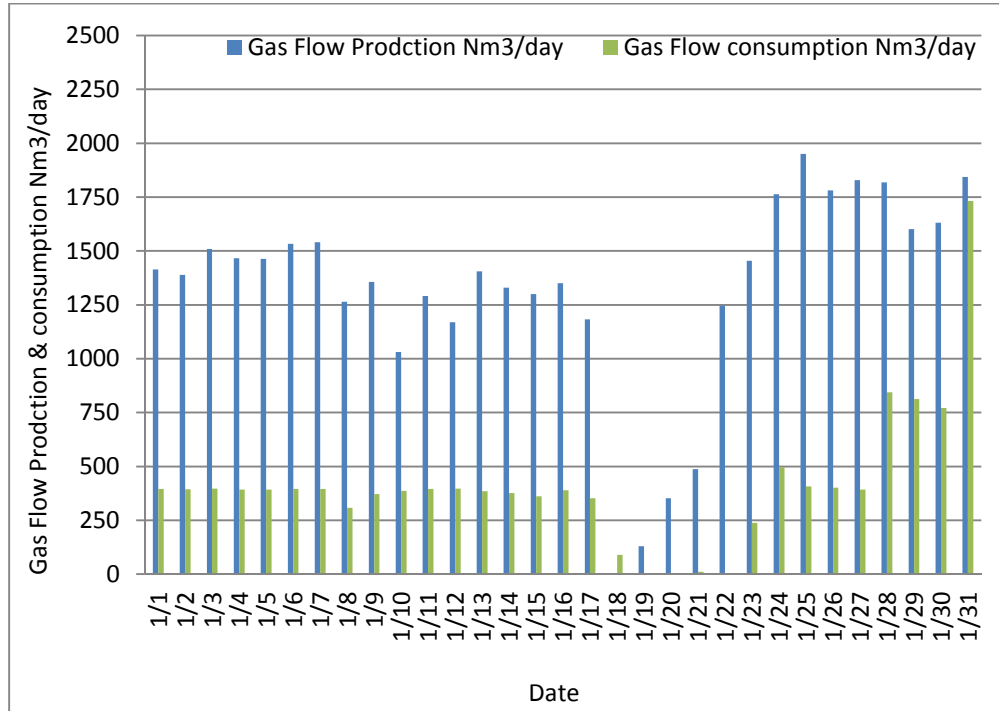
17: يوضح كمية الغاز الناتج والكمية المستهلكة لـ CHP لشهر والفرق بينهما والذي يتم استخدامه للبوليلر درجة حرارة الهاضم اللاهوائي
