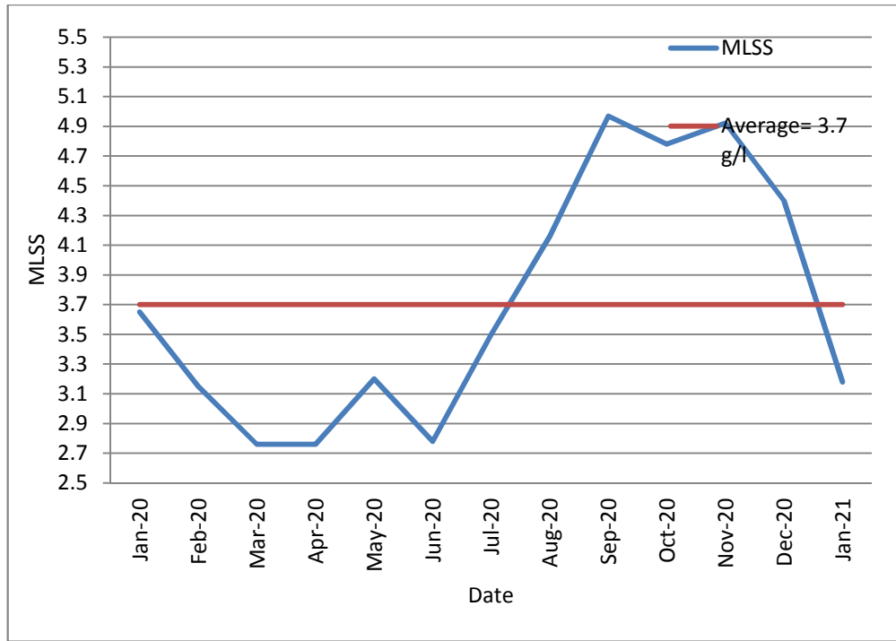
12: يوضح قيم نسبة المواد الصلبة المعلقة الحيوية في خزانات التهوية (MLSS) 2020/1 2021/1
