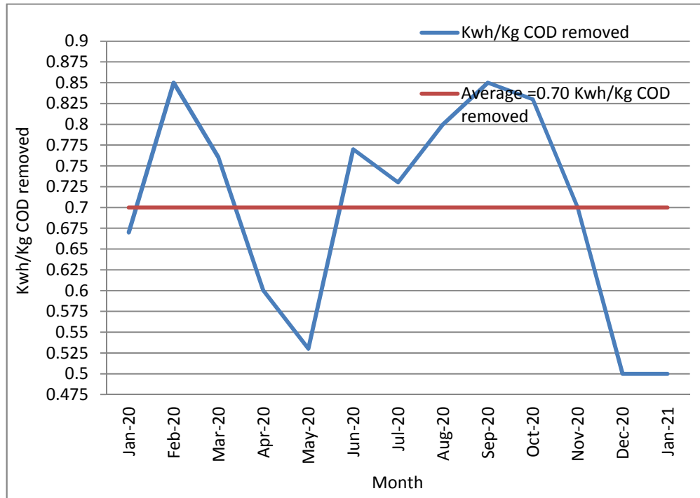
19: يوضح كميات الطاقة الكهربائية المستخدمة بدلالة كيلو واط ساعة لكل كغم COD 2021/1 2020/1
