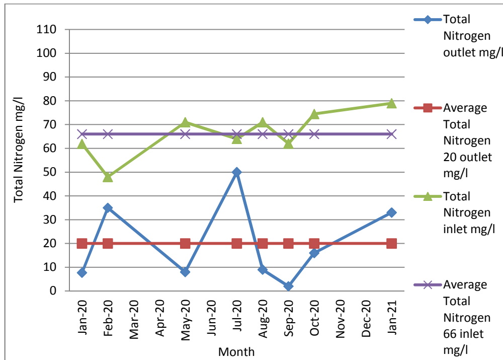
15: يبين فحوصات عملية إزالة النيتروجين 2020/1 2021/1 مع العلم بانه في شهور 3 4 6 11 12 لم يتم ( - )
