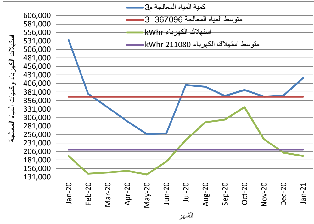
18: يوضح قيمة استهلاك الكهرباء وكمية المياه المعالجة 2021/1 2020/1
