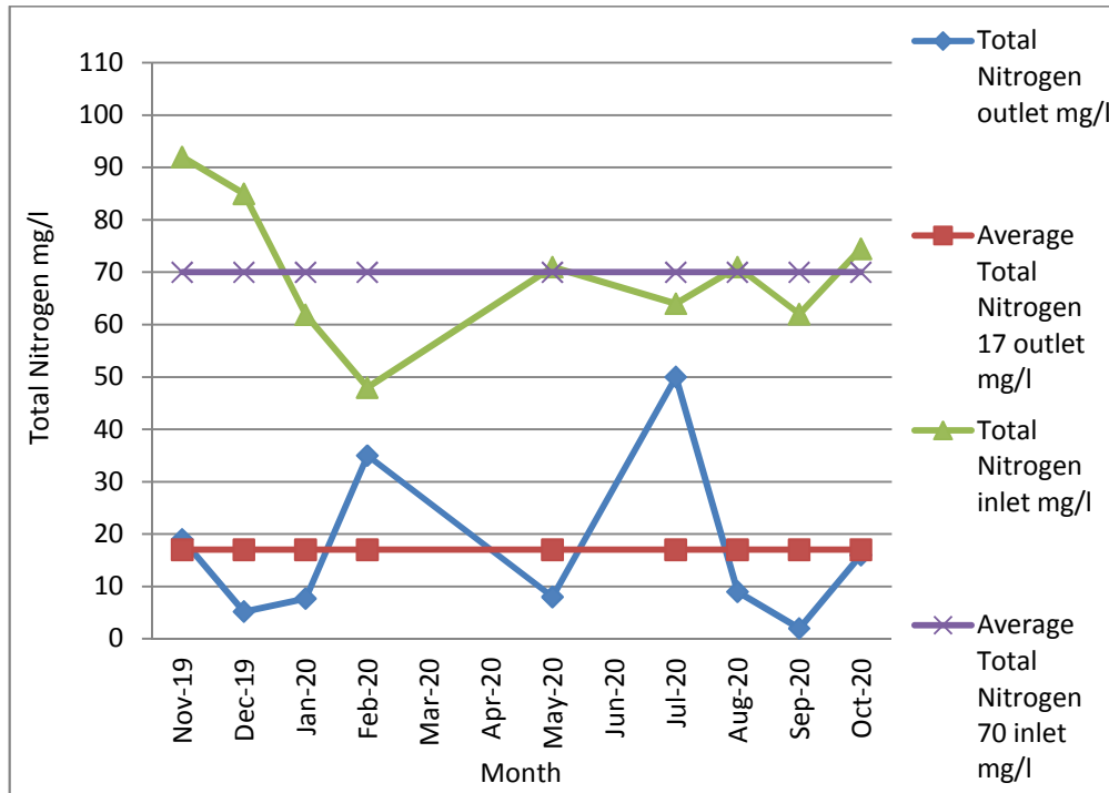
15: يبين فحوصات عملية إزالة النيتروجين 2019/12 مع العلم بانها في شهور 3 4 6 11 12 لم يتم ( - )
