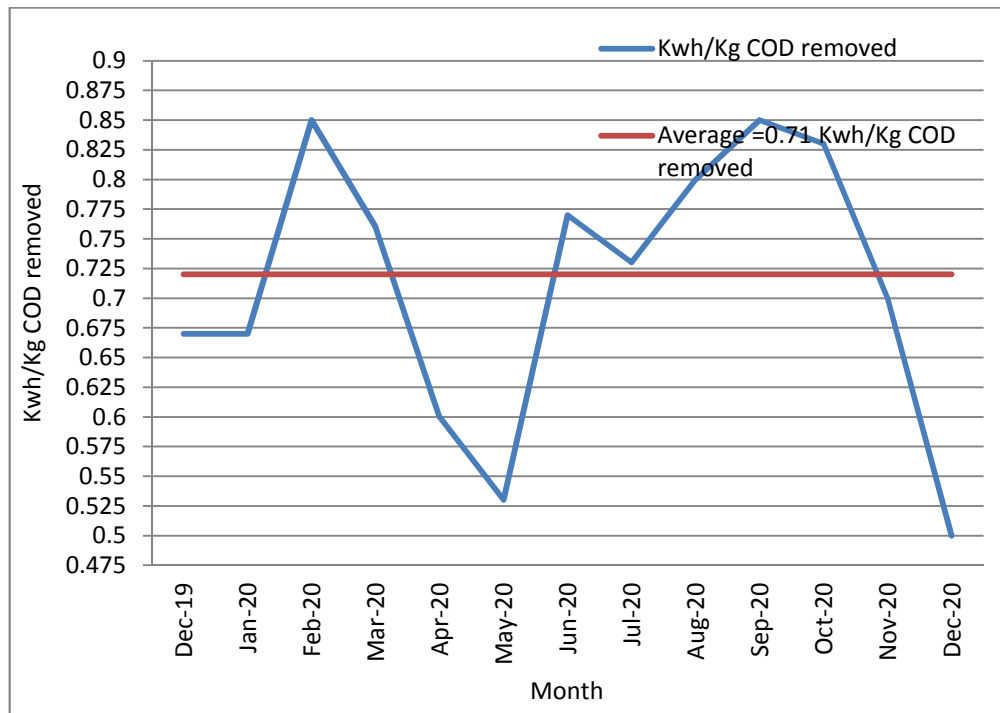
19: يوضح كميات الطاقة الكهربائية المستخدمة بدلالة كيلو واط ساعة لكل كغم COD 2020/12 2019/12
