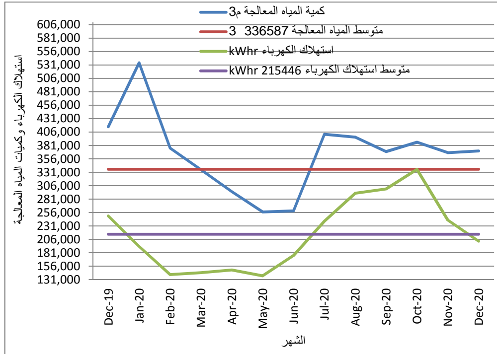
18: يوضح قيمة استهلاك الكهرباء وكمية المياه المعالجة 2020/12 2019/12
