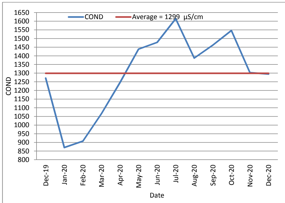
13 : يوضح قيم التوصيلية الكهربائية للمياه العادمة الداخلة (Conductivity) 2020/12 2019/12
