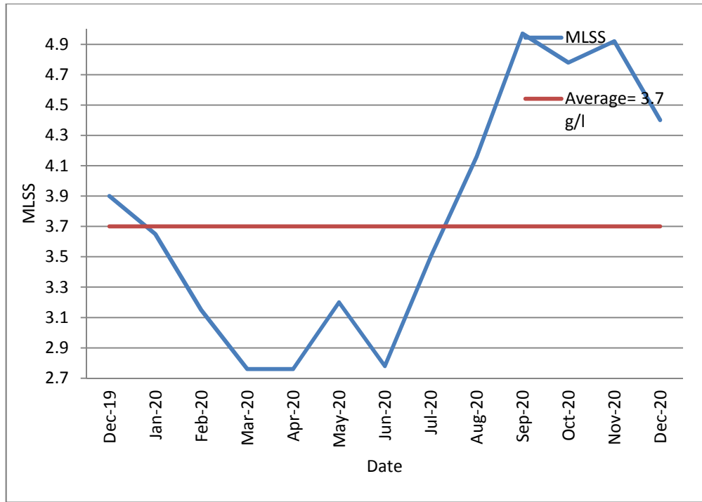
12: يوضح قيم نسبة المواد الصلبة المعقدة الحيوية في خزانات التهوية ( MLSS ) 2020/12 2019/12
