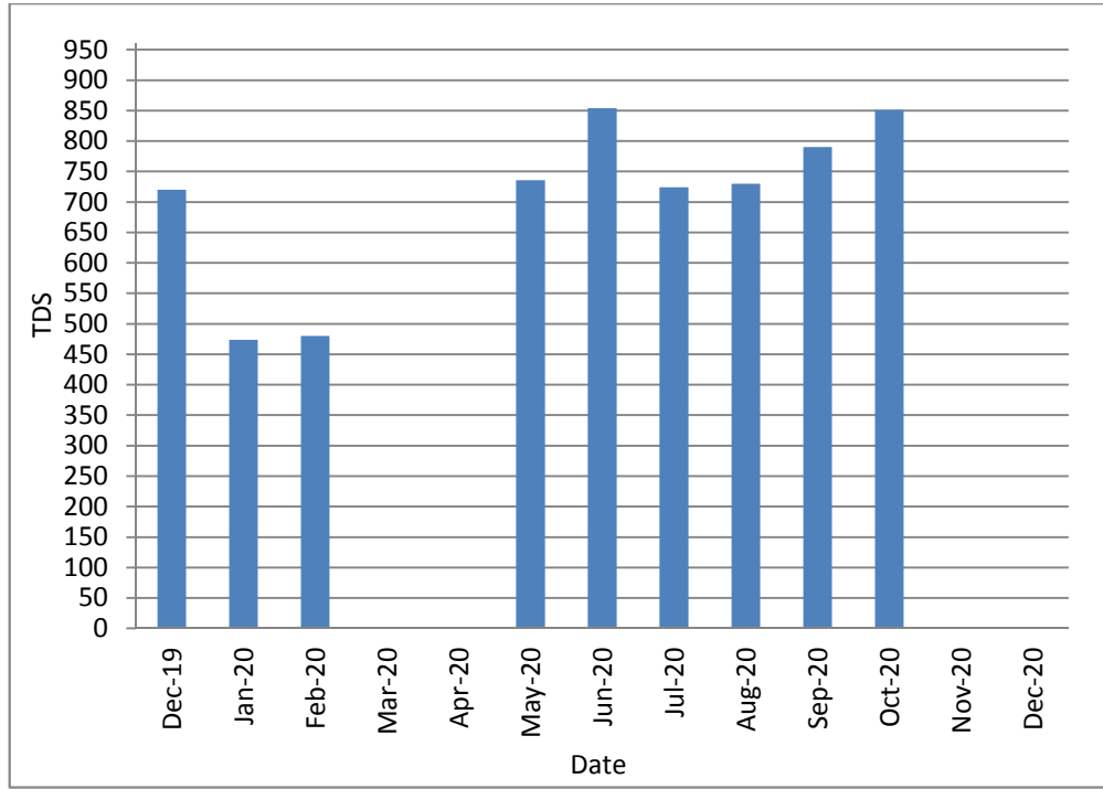
14: يوضح قيم نسبة الاملاح الكلية الذائبة في المياه المعالجة (TDS) 2019/12 مع العلم بانها في شهور 3 4 2020/12 لم يتم عمل فحص ( - )
