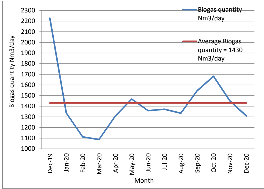
16: بوضوح الكميات المنتجة من الغاز الحيوي يومياً 2020/12 2019/12
