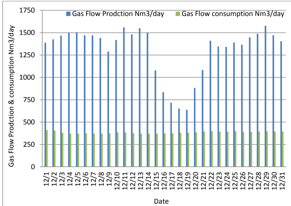
17: بوضوح كمية الغاز الناتج والكمية المستهلكة لـ CHP لشهر والفرق بينهما والذي يتم استخدامه للبوليلر درجة حرارة الهاضم اللاهوائي
