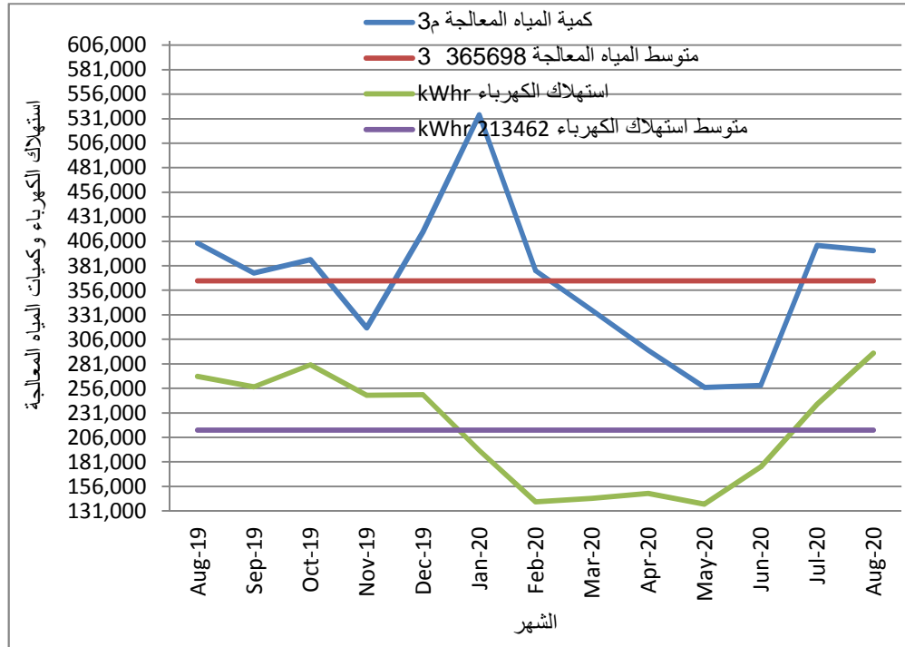
18: يوضح قيمة استهلاك الكهرباء وكمية المياه المعالجة 2020/8 2019/8
