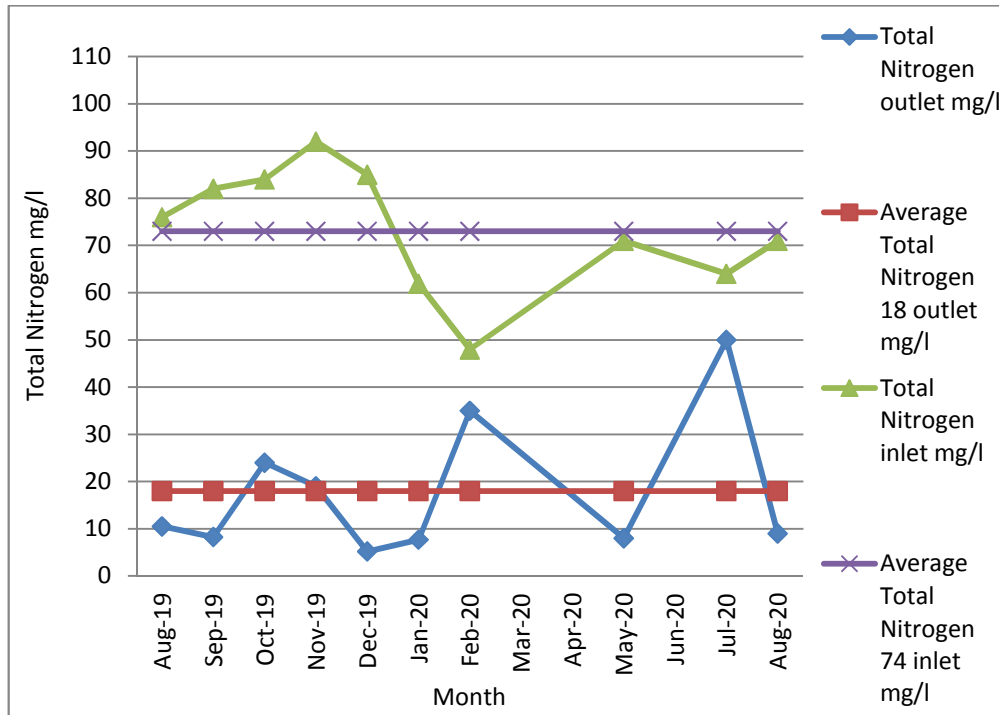
15: يبين فحوصات عملية إزالة النيتروجين 2019/8 مع العلم بانها في شهور 3 4 6 لم يتم ( - )
