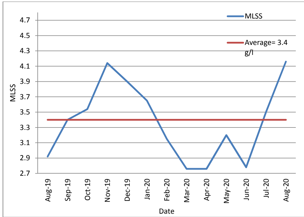
12: يوضح قيم نسبة المواد الصلبة المعلقة الحيوية في خزانات التهوية (MLSS) 2020/8 2019/8
