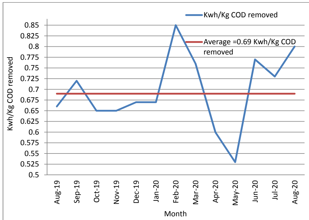
19: يوضح كميات الطاقة الكهربائية المستخدمة بدلالة كيلو واط ساعة لكل كغم COD 2020/8 2019/8
