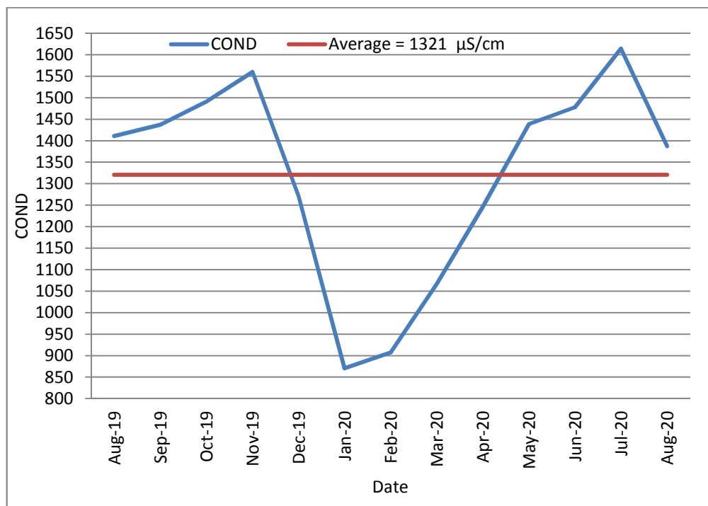
13 : يوضح قيم الموصلية الكهربائية (Conductivity) للمياه العادمة الداخلة 2020/8 2019/8
