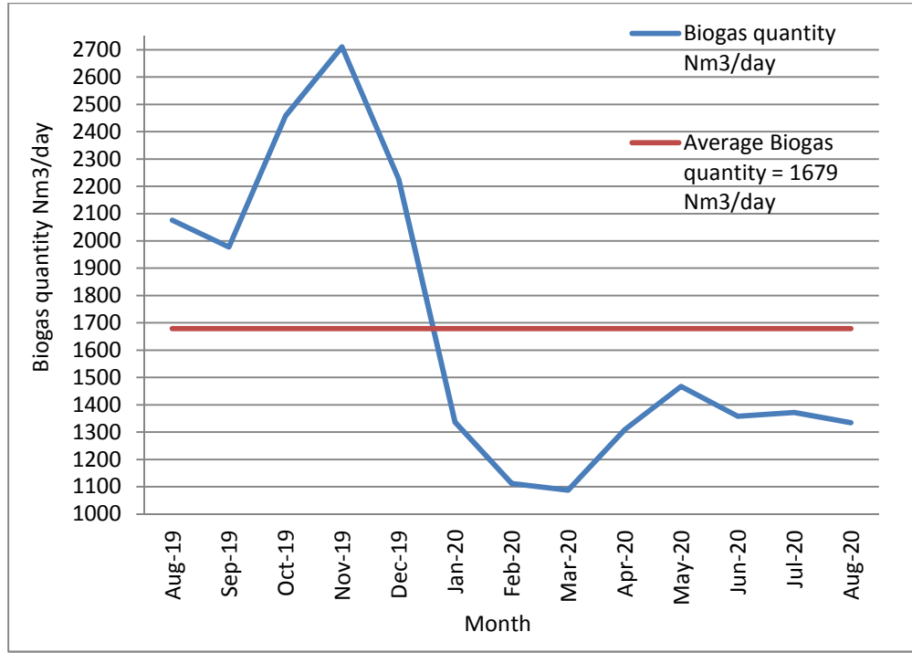
16: يوضح الكميات المنتجة من الغاز الحيوي يوميا ً 2020/8 2019/8
