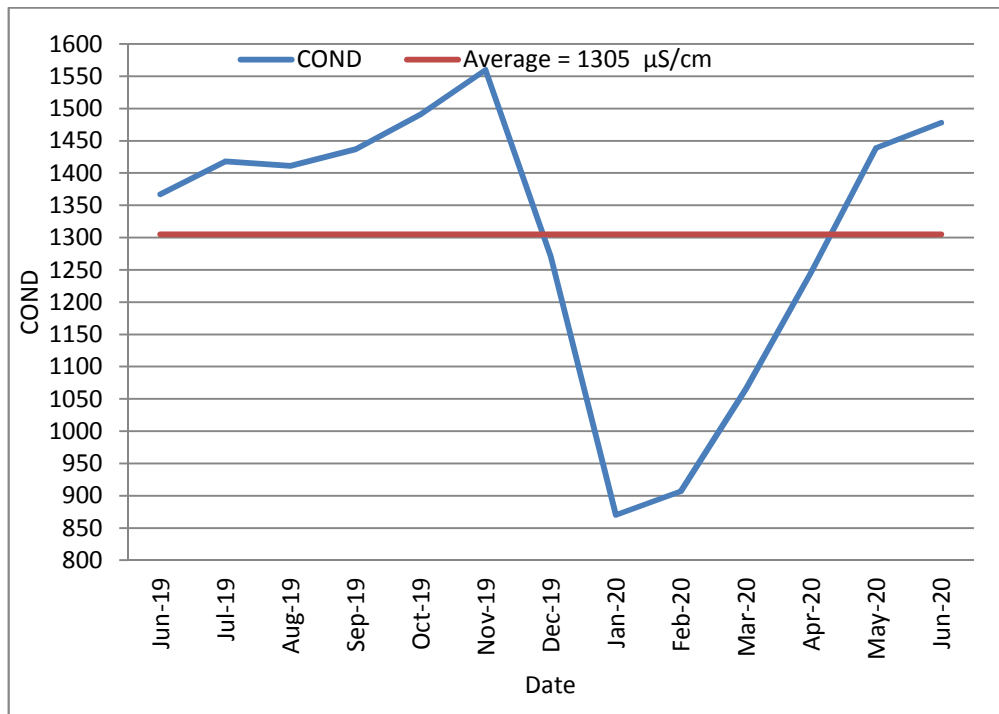
13 : يوضح قيم الموصلية الكهربائية (Conductivity) للمياه العادمة الداخلة 2020/6 2019/6
