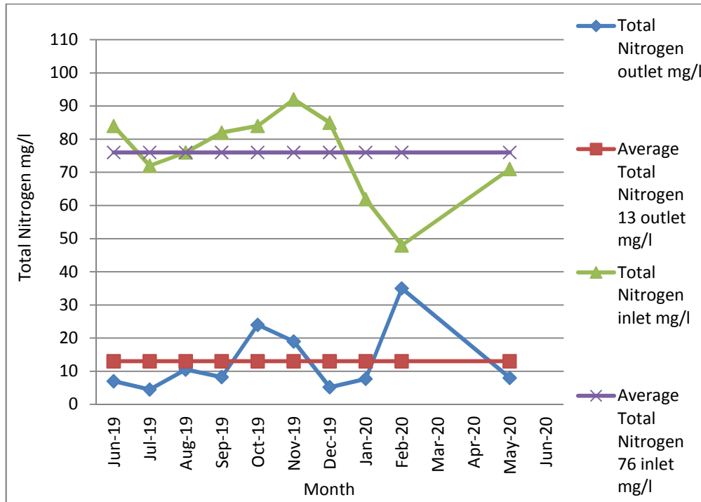
15: يبين فحوصات عملية إزالة النيتروجين 2019/6 مع العلم بانها في شهور 3 4 6 لم يتم ( - )
