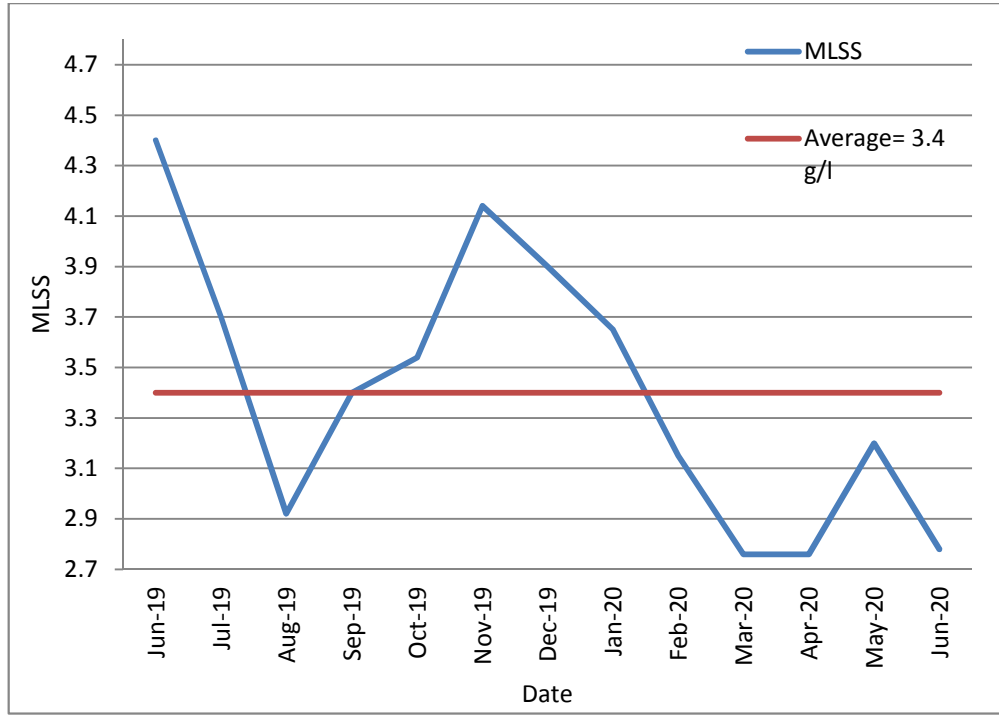
12: يوضح قيم نسبة المواد الصلبة المعقدة الحيوية في خزانات التهوية (MLSS) 2020/6 2019/6
