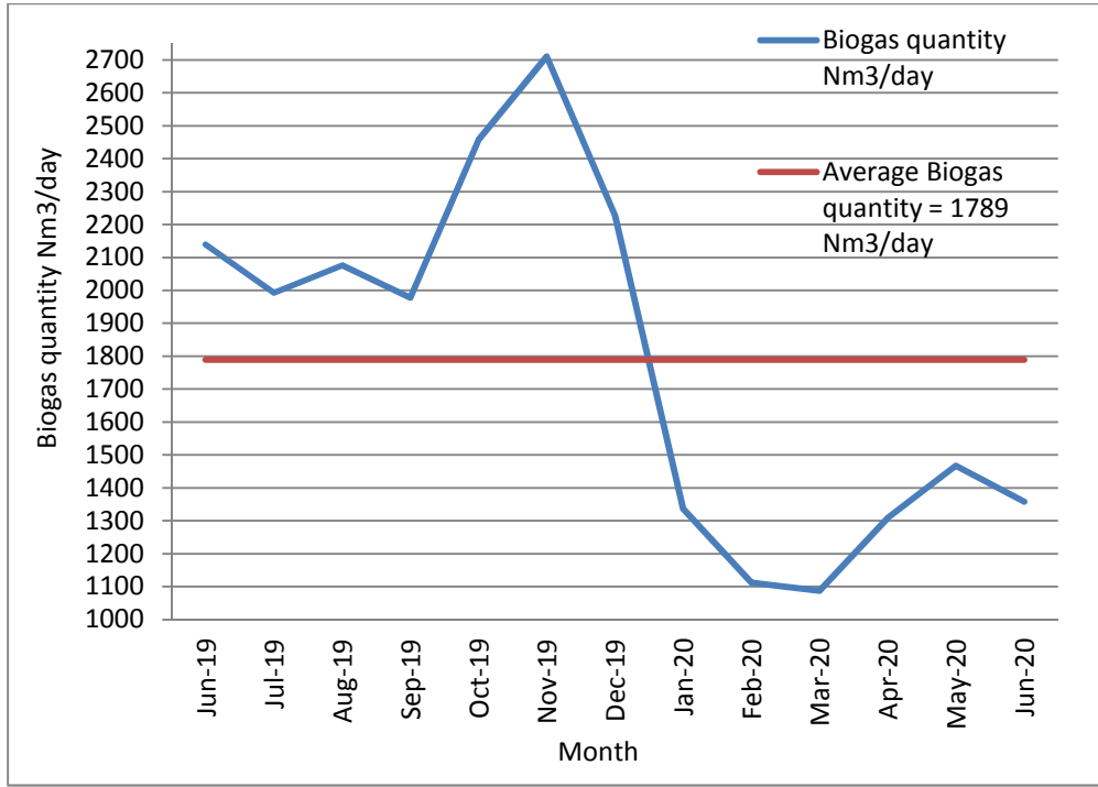
16: يوضح الكميات المنتجة من الغاز الحيوي يومياً 2020/6 2019/6
