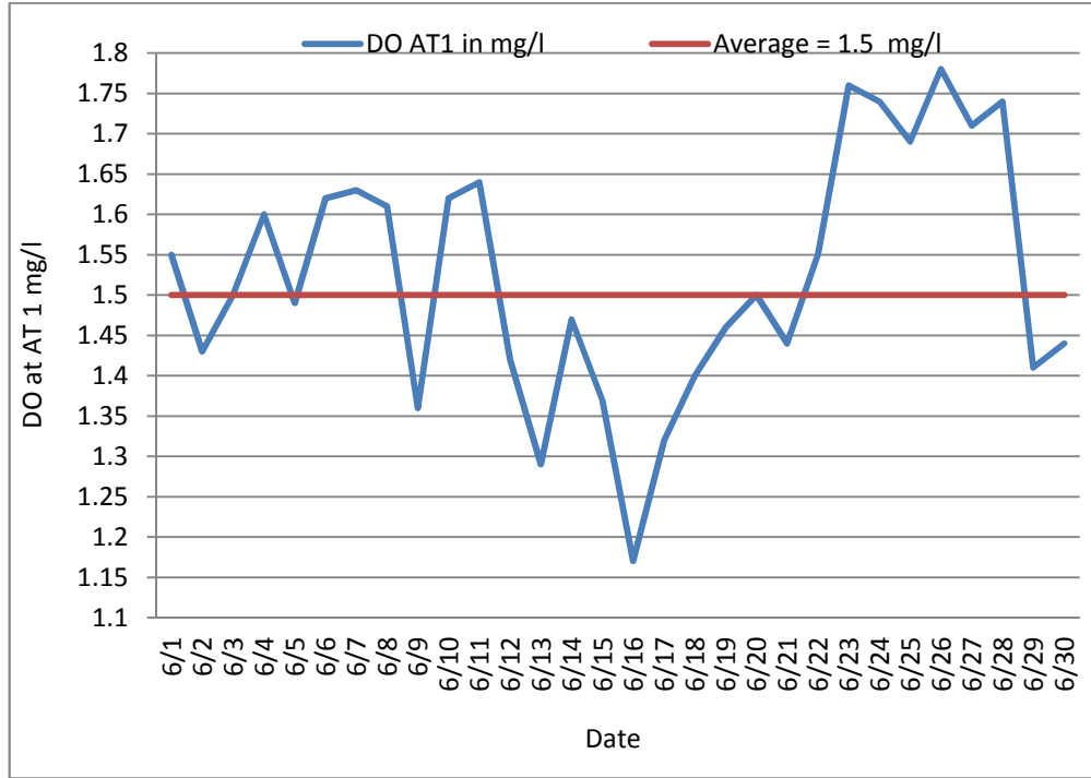
1 : يوضح تركيز الأوكسجين المذاب في خزان التهويه
