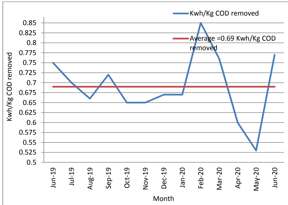
19: يوضح كميات الطاقة الكهربائية المستخدمة بدلالة كيلو واط ساعة لكل كغم COD 2020/6 2019/6
