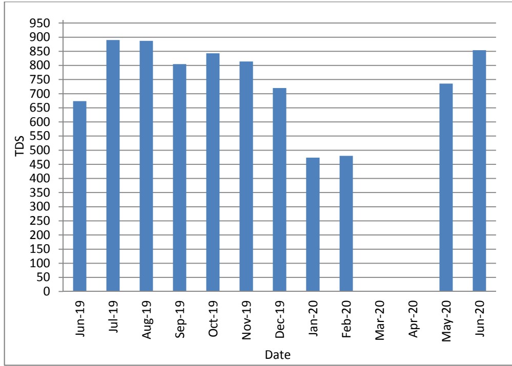
14: يوضح قيم نسبة الاملاح الكلية الذائبة في المياه المعالجة (TDS) 2019/6 مع العلم بانها في شهر 3 2020/6 لم يتم عمل فحص ( - )
