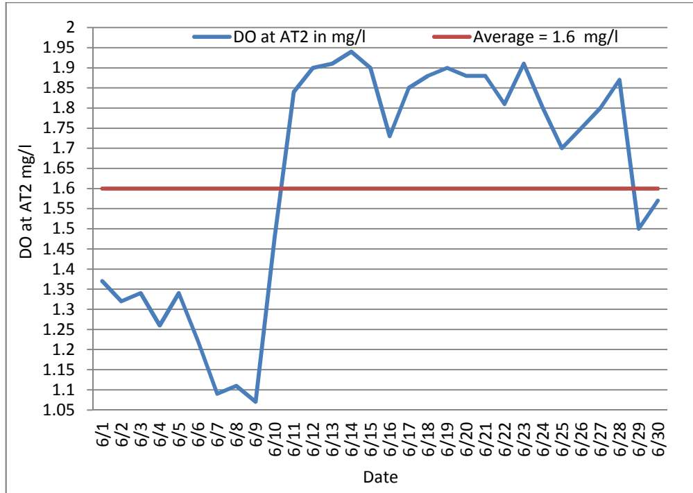
2 : يوضح تركيز الأوكسجين المذاب في خزان التهويه
