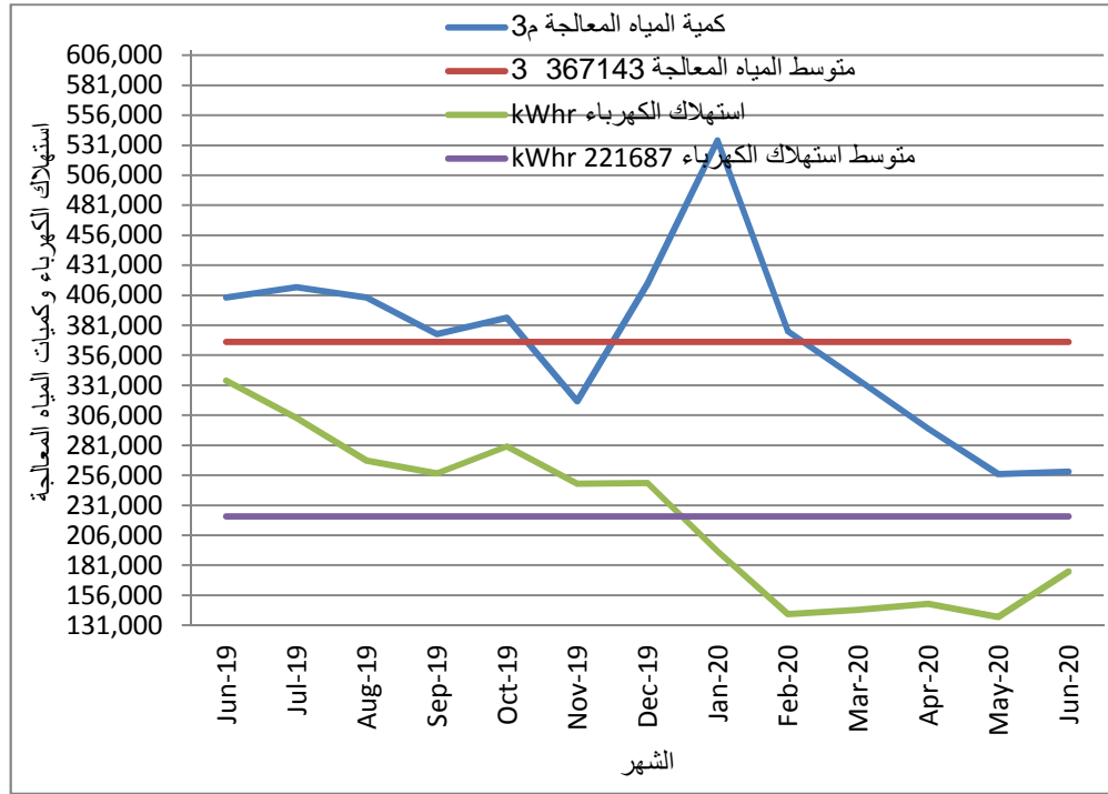
18: يوضح قيمة استهلاك الكهرباء وكمية المياه المعالجة 2020/6 2019/6
