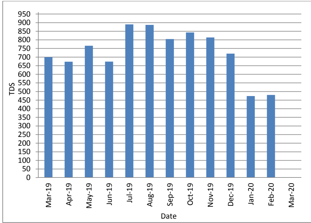
14: يوضح قيم نسبة الاملاح الكلية الذائبة في المياه المعالجة (TDS) 2019/3 مع العلم بانها في شهر 3 لم يتم 2020/3
