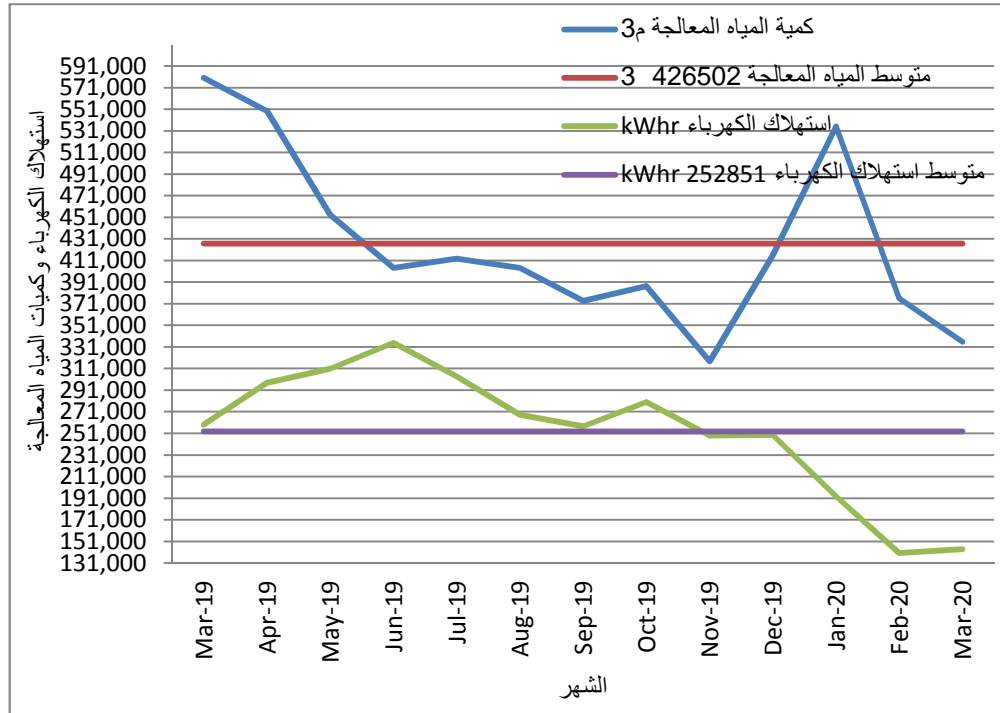
18: يوضح قيمة استهلاك الكهرباء وكمية المياه المعالجة 2020/3 2019/3
