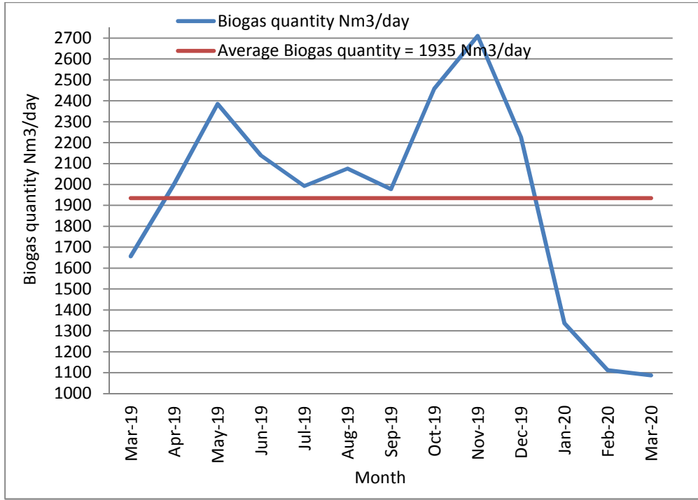
16: يوضح الكميات المنتجة من الغاز الحيوي يوميا 2020/3 2019/3
