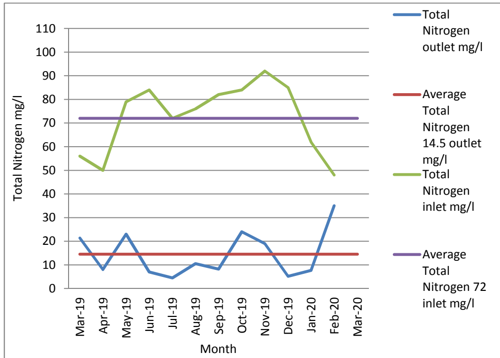
15: يبين فحوصات عملية إزالة النيتروجين 2019/3 مع العلم بانها في شهر 3 لم يتم فحص 2020/3
