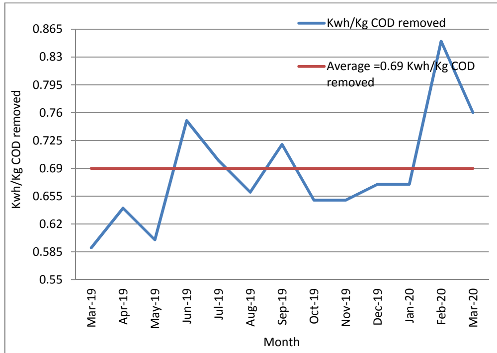
19: يوضح كميات الطاقة الكهربائية المستخدمة بدلالة كيلو واط ساعة لكل كغم COD 2020/3 2019/3
