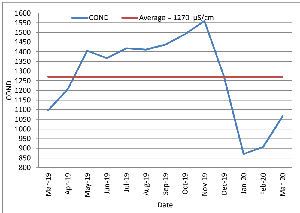
13 : يوضح قيم الموصلية الكهربائية (Conductivity) للمياه العادمة الداخلة 2020/3 2019/3
