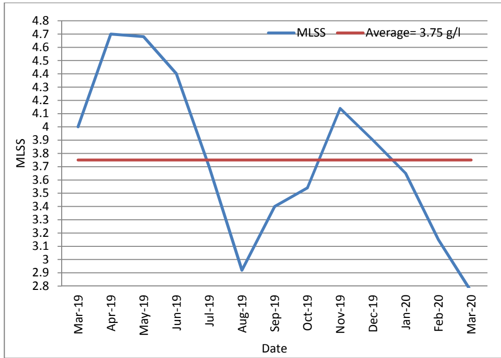
12: يوضح قيم نسبة المواد الصلبة المعلقة الحيوية في خزانات التهوية (MLSS) 2020/3 2019/3
