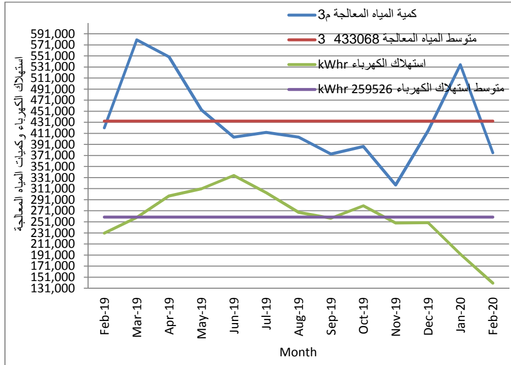
18: يوضح قيمة استهلاك الكهرباء وكمية المياه المعالجة 2020/2 2019/2
