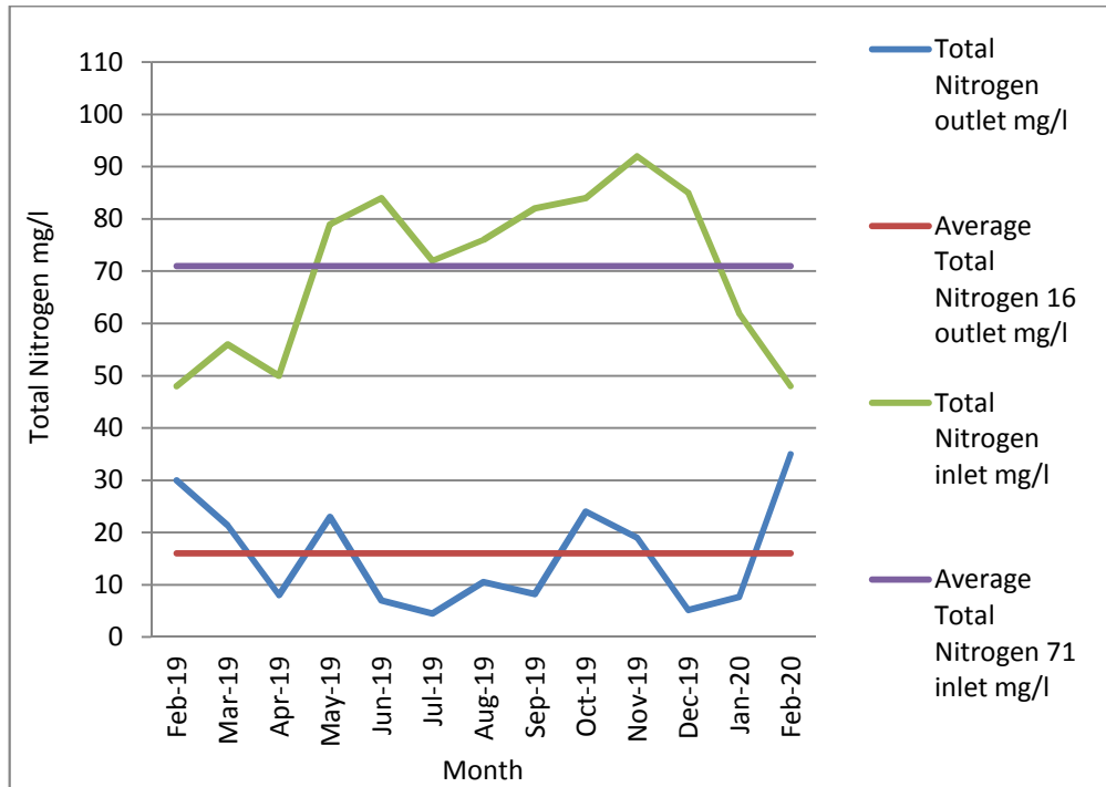
15: يبين فحوصات عملية إزالة النيتروجين 2020/2 2019/2
