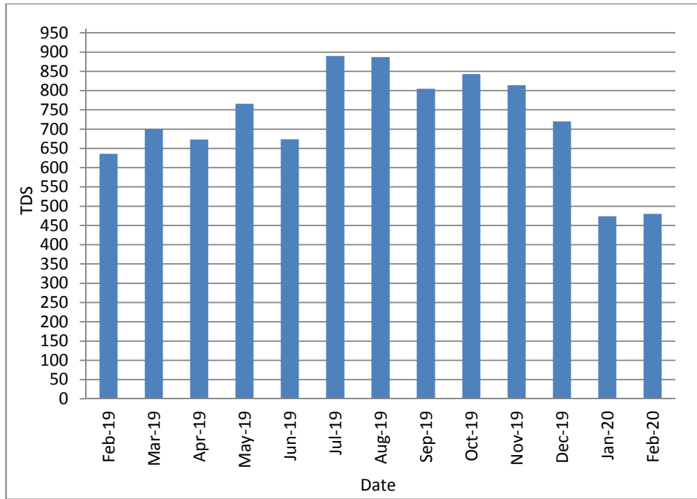
14: يوضح قيم نسبة الاملاح الكلية الذائبة في المياه المعالجة (TDS) 2020/2 2019/2
