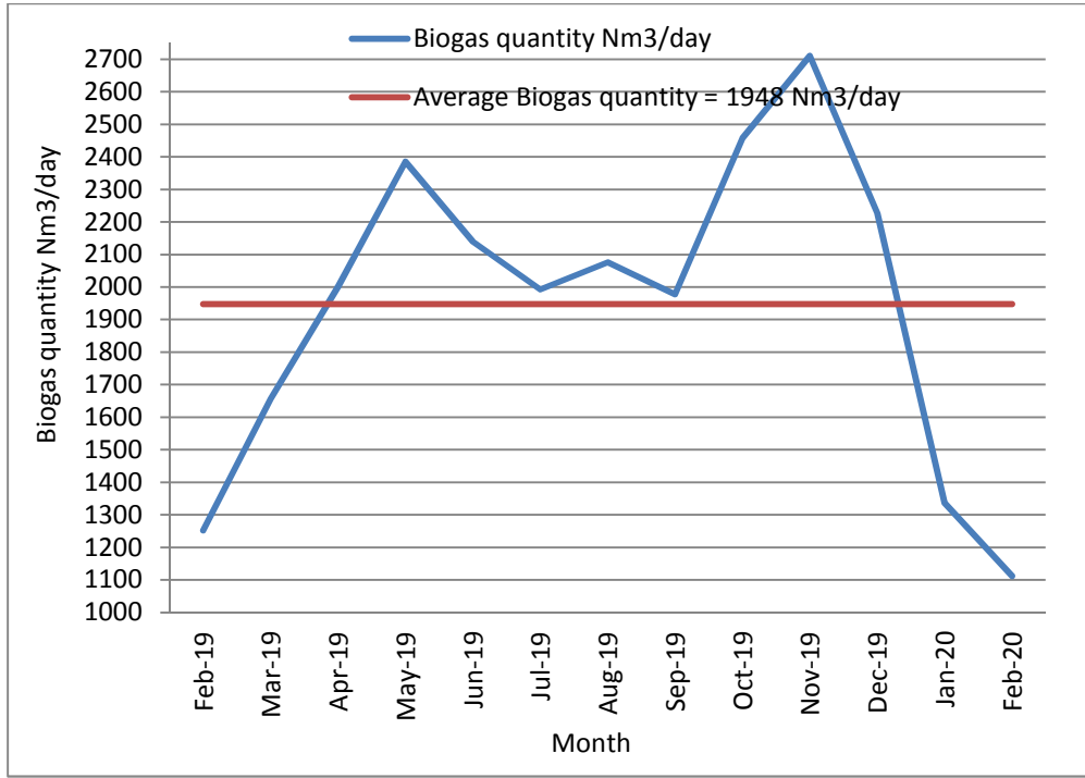
16: يوضح الكميات المنتجة من الغاز الحيوي يوميا 2020/2 2019/2
