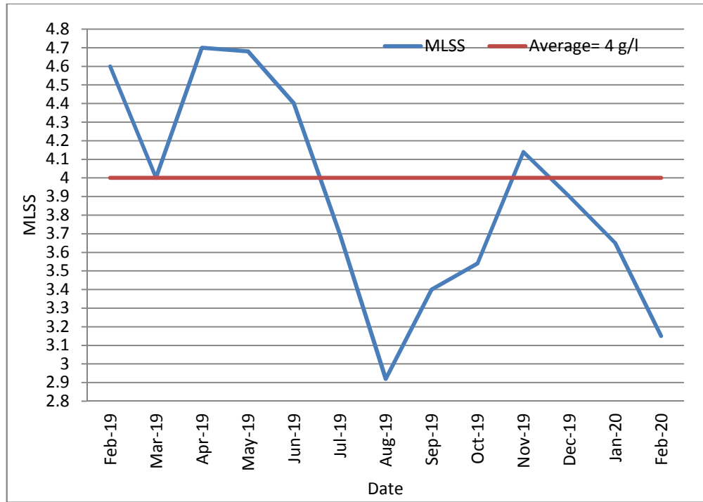
12: يوضح قيم نسبة المواد الصلبة المعلقة الحيوية في خزانات التهوية (MLSS) 2020/2 2019/2
