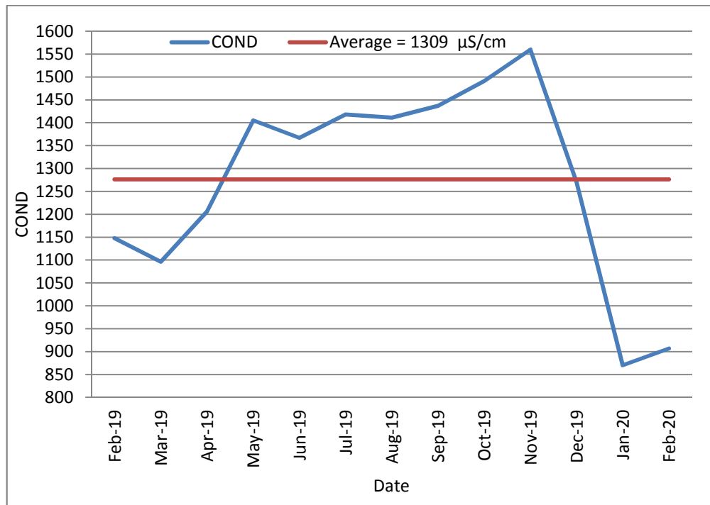
13 : يوضح قيم الموصلية الكهربائية (Conductivity) للمياه العادمة الداخلة 2020/2 2019/2
