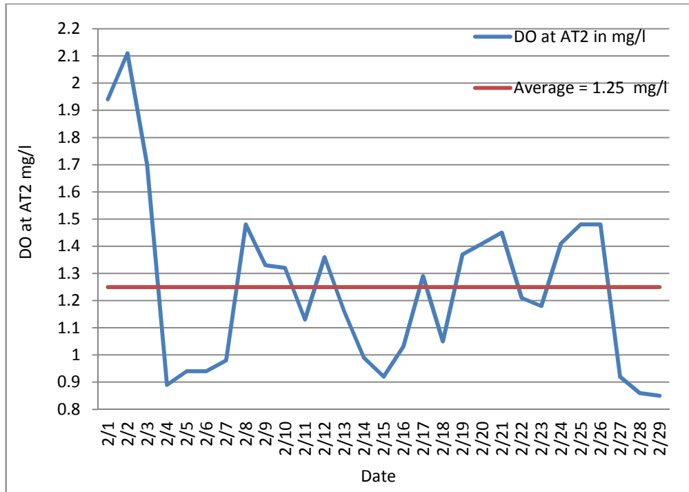
2 : يوضح تركيز الأوكسجين المذاب في خزان التهويه
