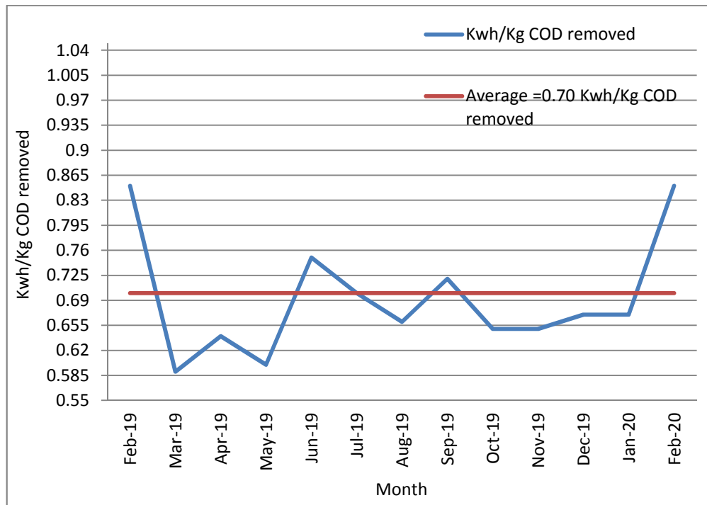
19: يوضح كميات الطاقة الكهربائية المستخدمة بدلالة كيلو واط ساعة لكل كغم COD 2020/2 2019/2
