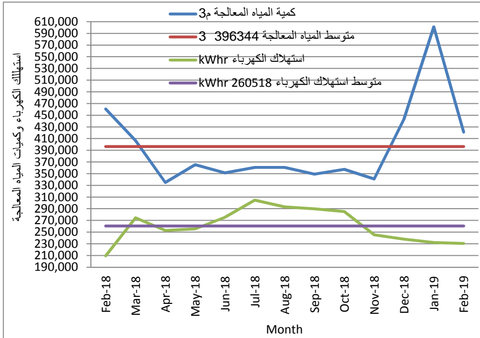
18: يوضح قيمة استهلاك الكهرباء وكمية المياه المعالجة 2018/2 2019/2
