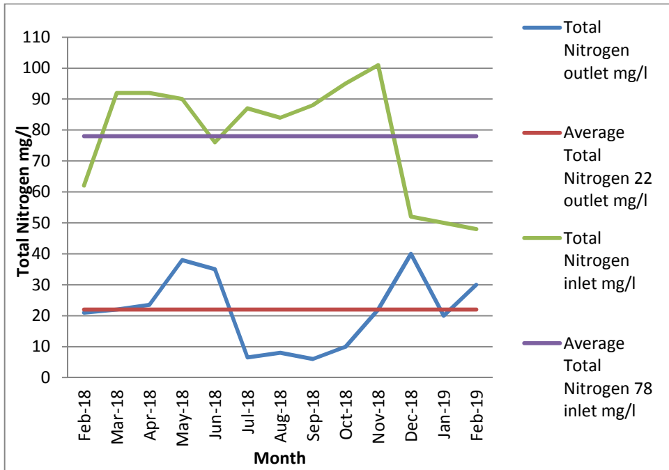
15: يبين فحوصات عملية إزالة النيتروجين 2018/2 2019/2
