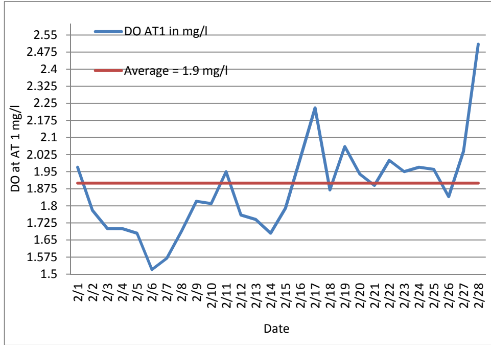
1 : يوضح الأوكسجين المذاب في خزان التهويه
