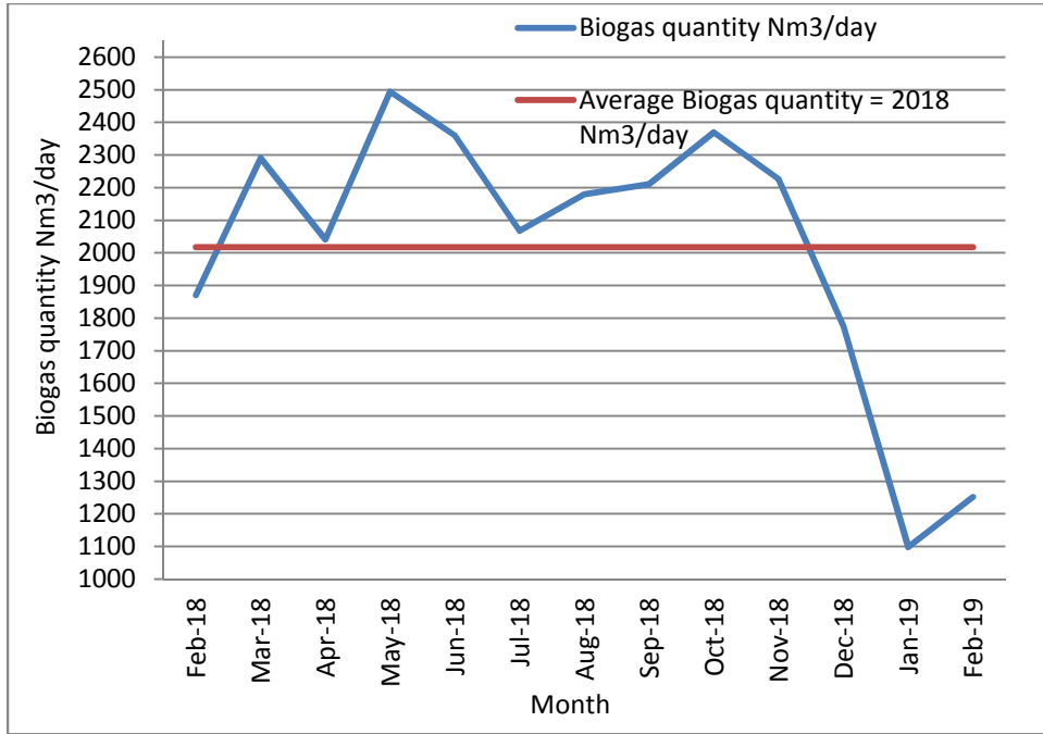
16: يوضح الكميات المنتجة من الغاز الحيوي يومياً من شهر 2018/2 2019/2
