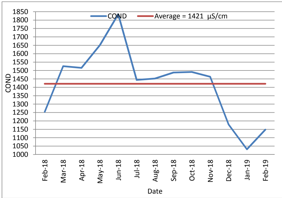
13 : يوضح قيم الموصلية الكهربائية (Conductivity) للمياه العادمة الداخلة 2018/2 2019/2
