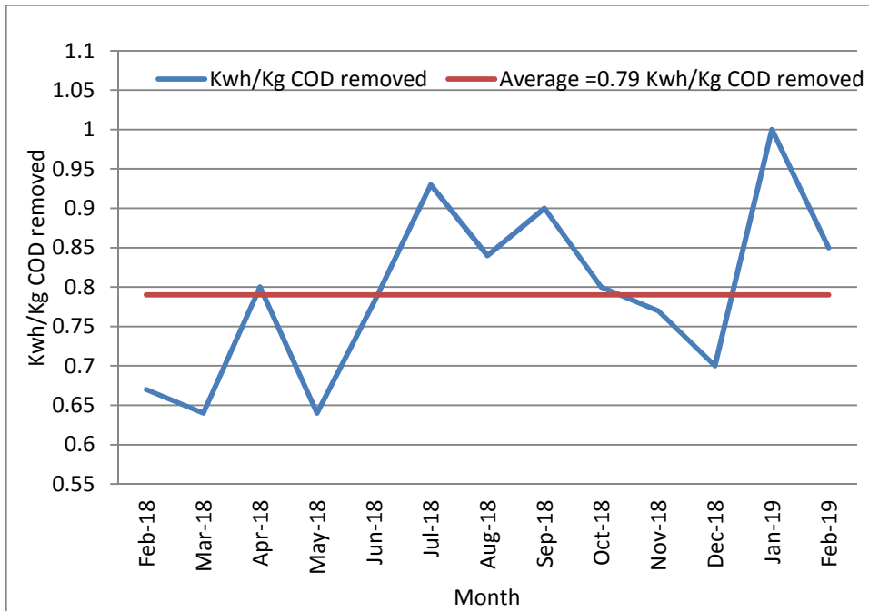
19: يوضح كميات الطاقة الكهربائية المستخدمة بدلالة كيلو واط ساعة لكل كغم COD 2018/2 2019/2
