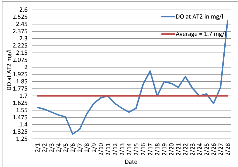
2 : يوضح الأوكسجين المذاب في خزان التهويه
