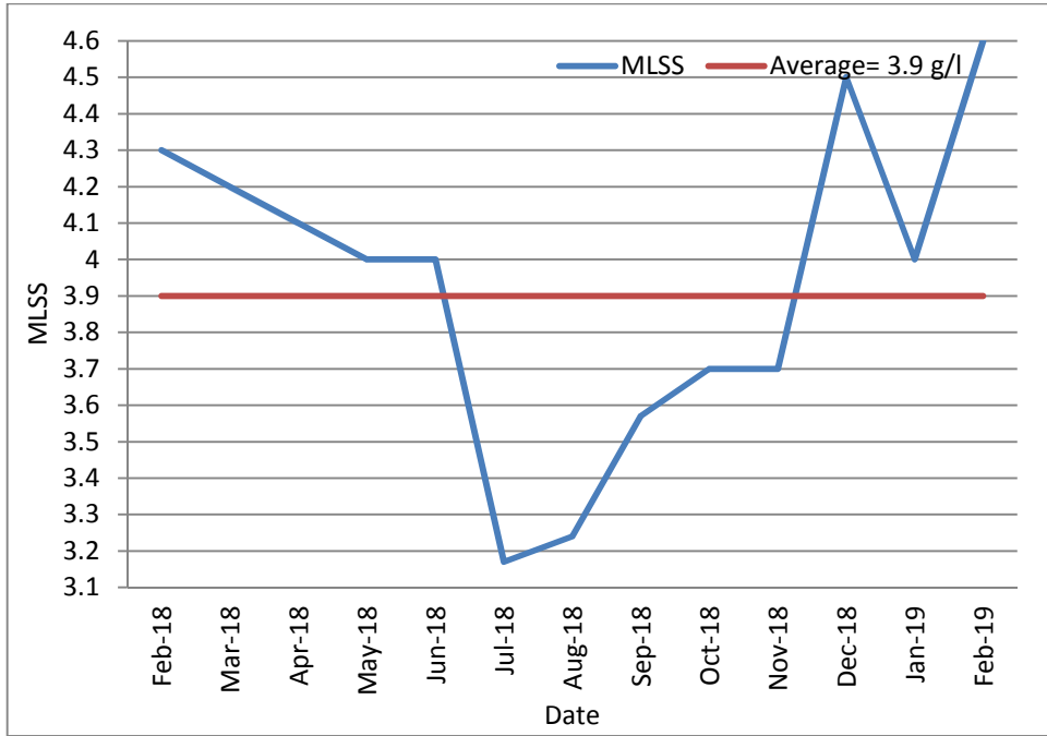
12: يوضح قيم نسبة المواد الصلبة المعلقة الحبيبية في خزانات التهوية (MLSS) 2018/2 2019/2
