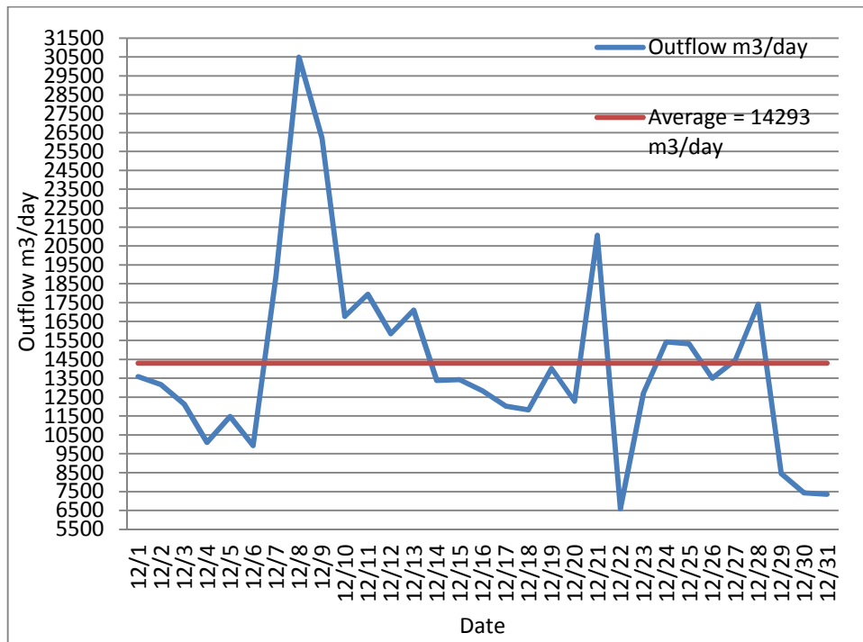
3 : بين كمية المياه المعالجة الخارجة يوميا من المحط .
