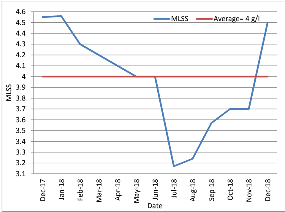
12: يوضح قيم نسبة المواد الصلبة المعلقة الحيوية في خزانات التهوية (MLSS) 2017/12 2018/12
