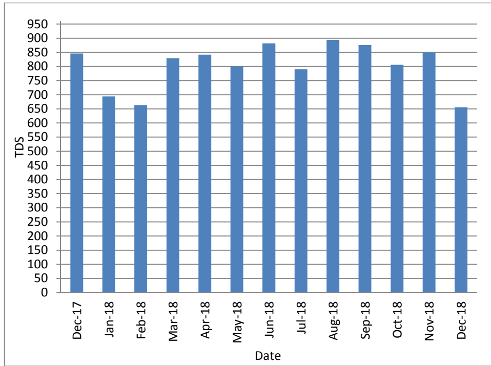
14: يوضح قيم نسبة الاملاح الكلية الذائبة في المياه المعالجة (TDS) 2017/12 2018/12
