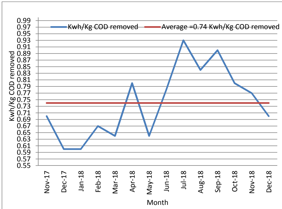
19: يوضح كميات الطاقة الكهربائية المستخدمة بدلالة كيلو واط ساعة لكل كغم COD 2018/12 2017/12
