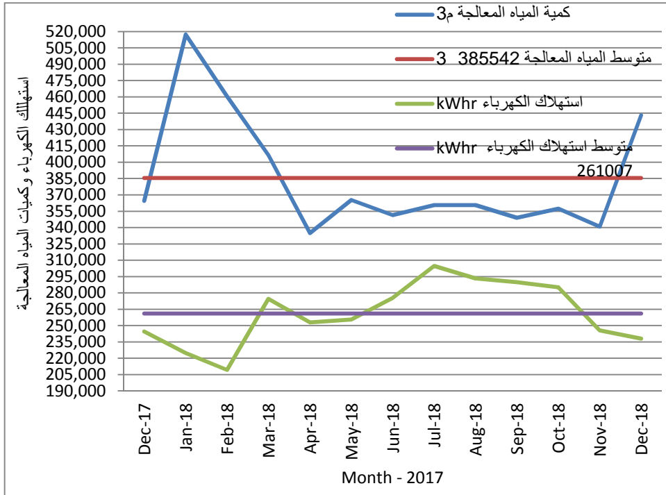
18: يوضح قيمة استهلاك الكهرباء وكمية المياه المعالجة 2018/12 2017/12
