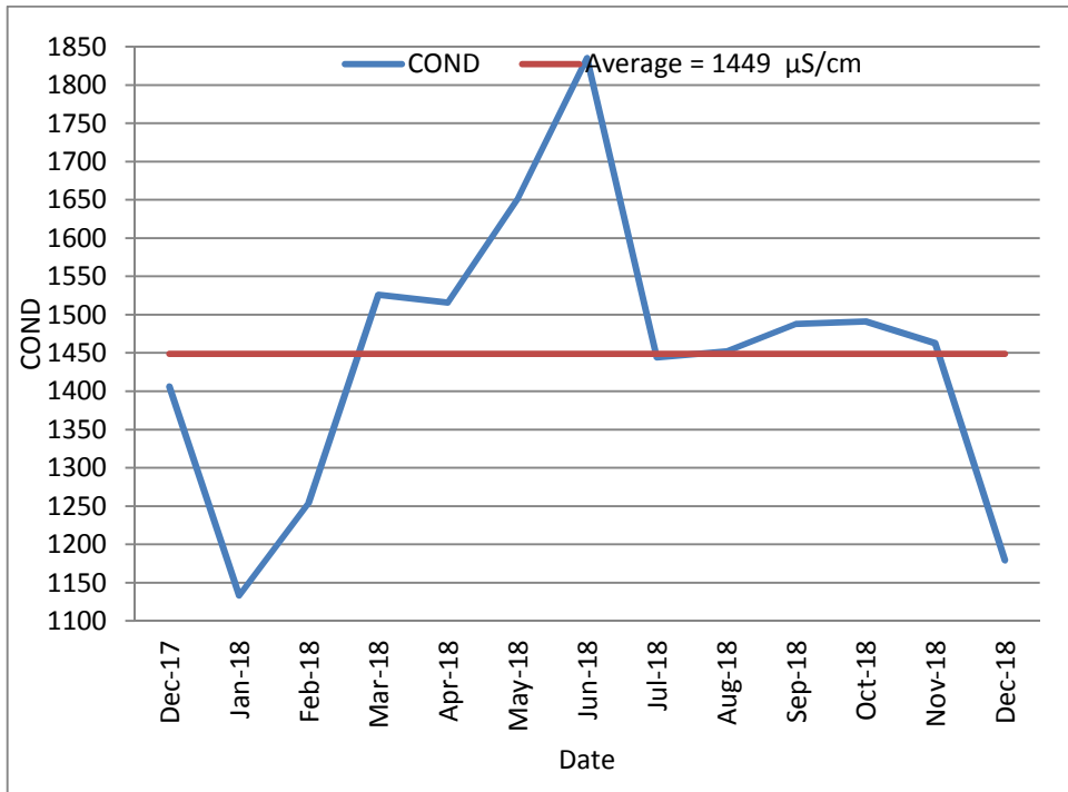
13 : يوضح قيم الموصلية الكهربائية للمياه العادمة الداخلة (Conductivity) 2017/12 2018/12
