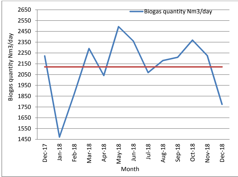
16: يوضح الكميات المنتجة من الغاز الحيوي يومياً من شهر 2017/12 2018/12
