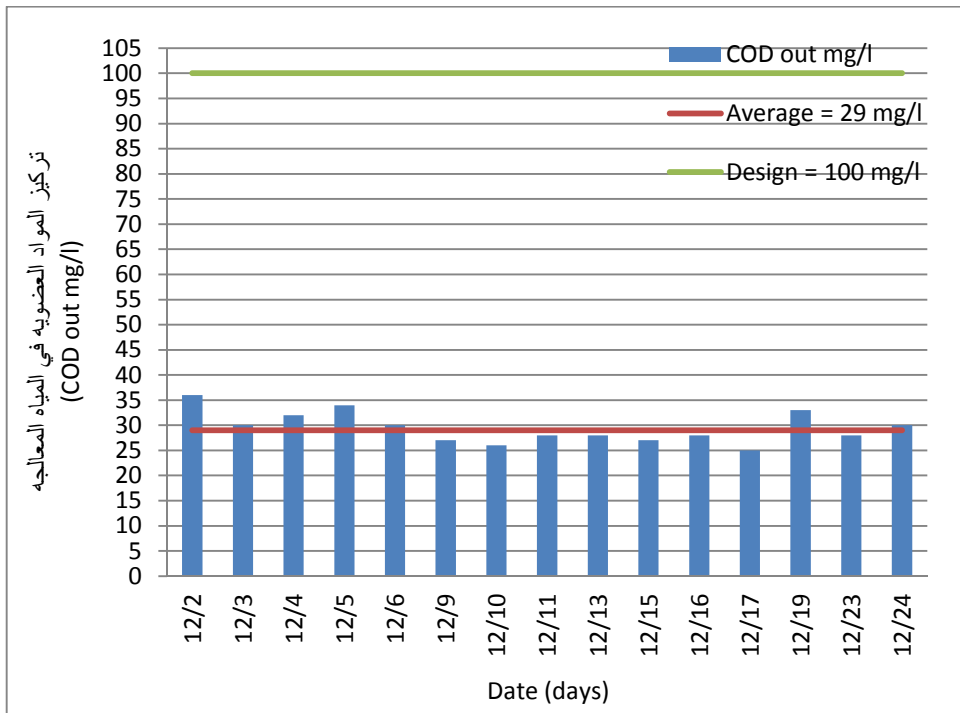
6 : يبين نتائج فحص تركيز المواد العضوية (COD in )
