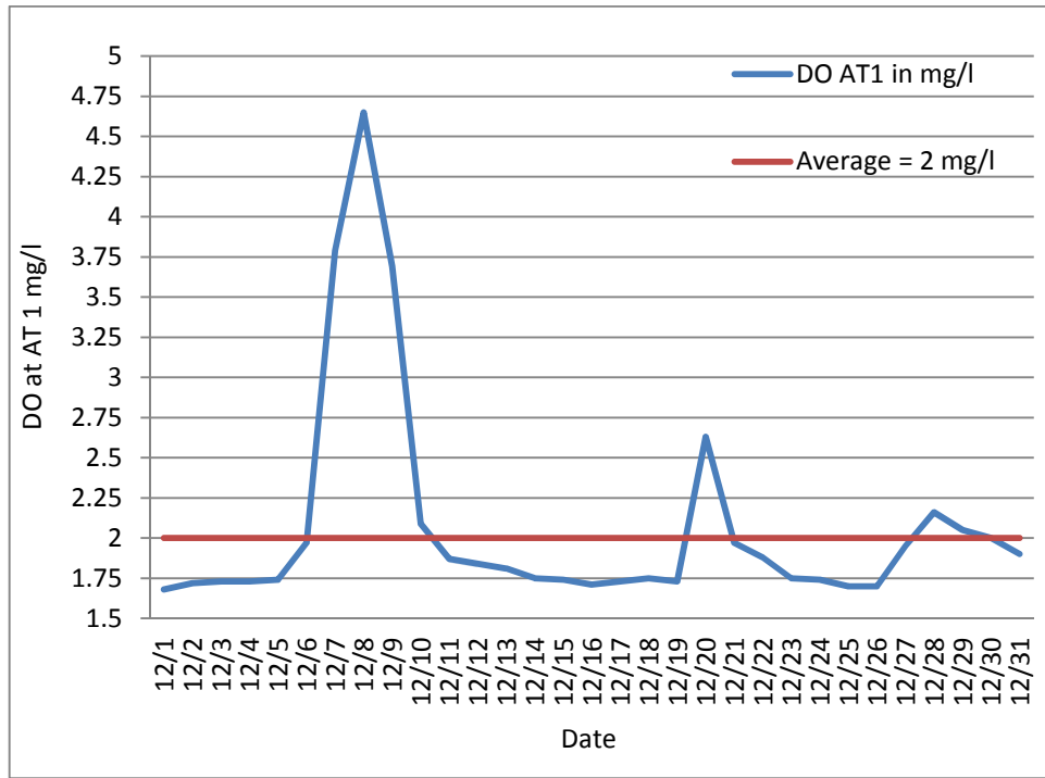
4 : يوضح الأكسجين المذاب في خزان التهوية 1
