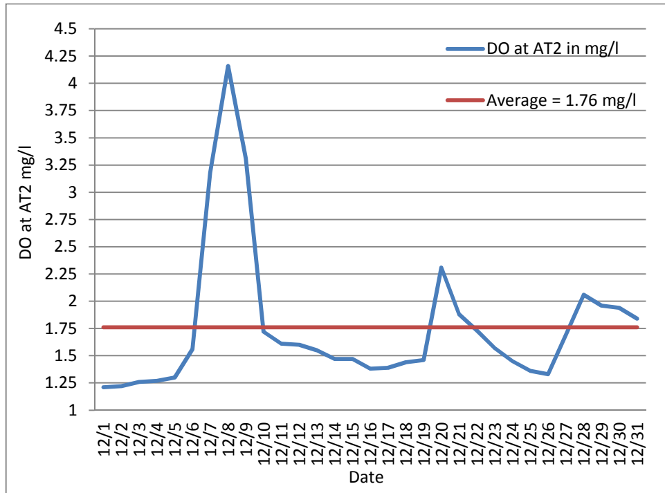
5 : يوضح الأكسجين المذاب في خزان التهوية 2
