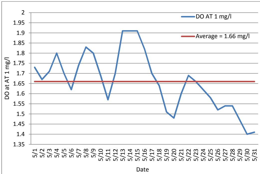
4 : يوضح الأكسجين المذاب في خزان التهوية 1
