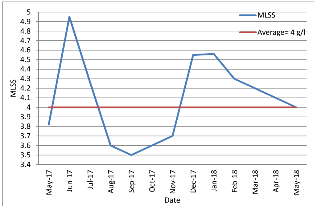
12: يوضح قيم نسبة المواد الصلبة المعلقة الحيوية في خزانات التهوية (MLSS) 2017/5 2018/5
