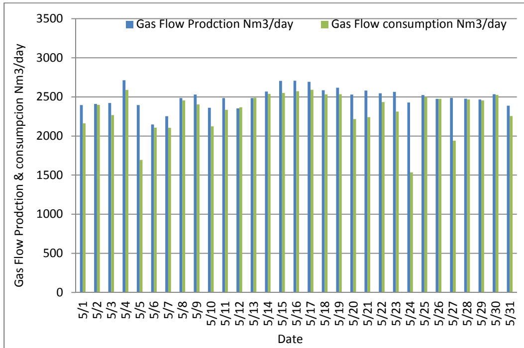
17: يوضح كمية الغاز الناتج والكمية المستهلكة لـ CHP لشهر ايار والفرق بينهما والذي يتم استخدامه للبولير لرفع درجة حرارة الهاضم اللاهوائي
