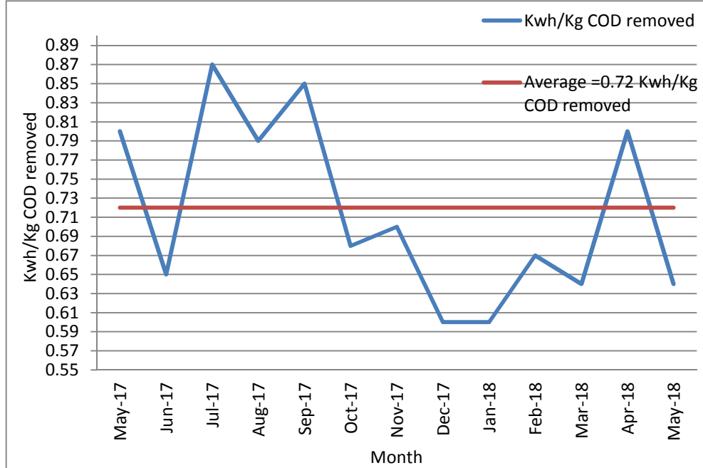
19: يوضح كميات الطاقة الكهربائية المستخدمة بدلالة كيلو واط ساعة لكل كغم COD 2018/5 2017/5
