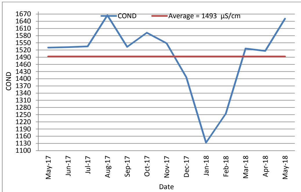
13 : يوضح قيم الموصلية الكهربائية (Conductivity) للمياه العادمة الداخلة 2017/5 2018/5
