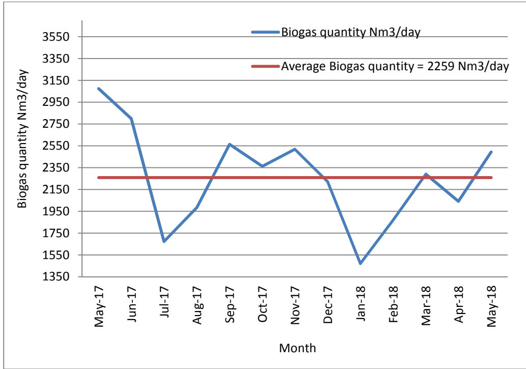
16: يوضح الكميات المنتجة من الغاز الحيوي يومياً من شهر 2017/5 إلى 2018/5
