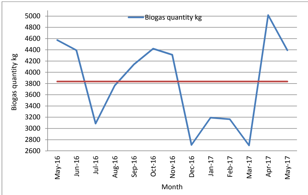
(11) : الكميات للغاز الحيوي /يوم
