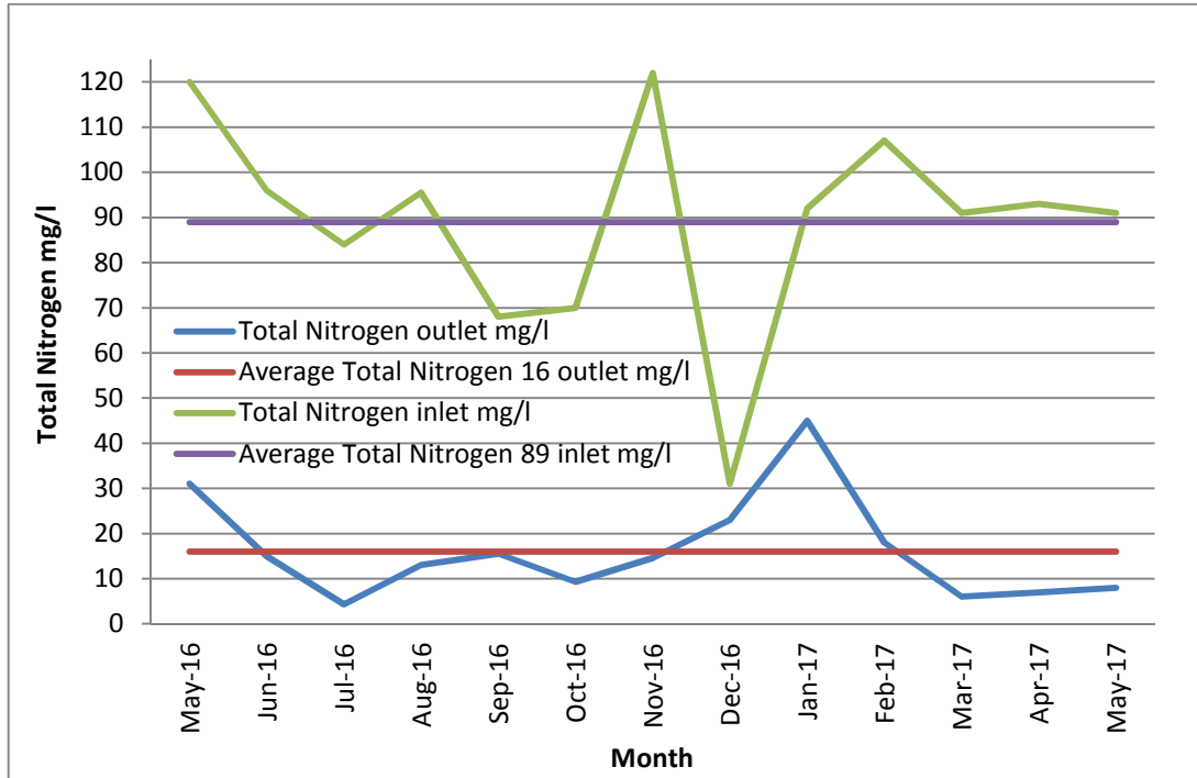
(20) : قيم الفحوصات الخاصة بعملية ازالة النيتروجين
