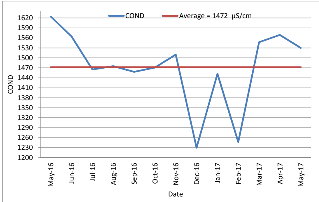
(16) : معدل قيم الموصلية الكهربائية الشهري للمياه العادمة الداخلة لمحطة المعالجة
