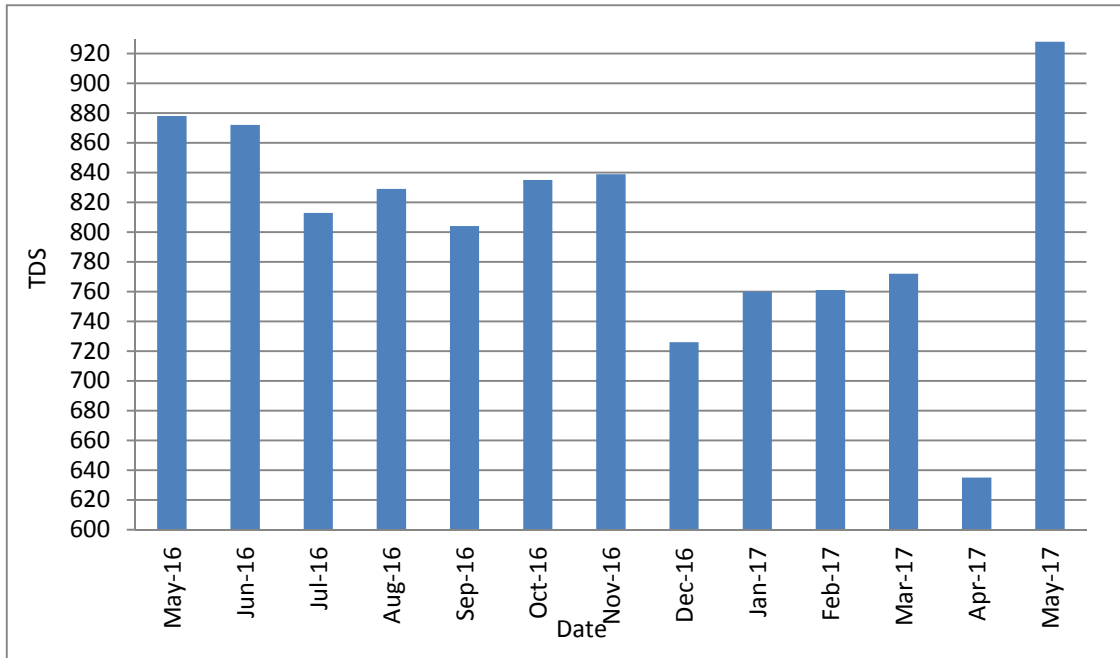
(17) : بعض القيم الناتجة عن تحليل الأملاح الذائبة للمياه المعالجة
