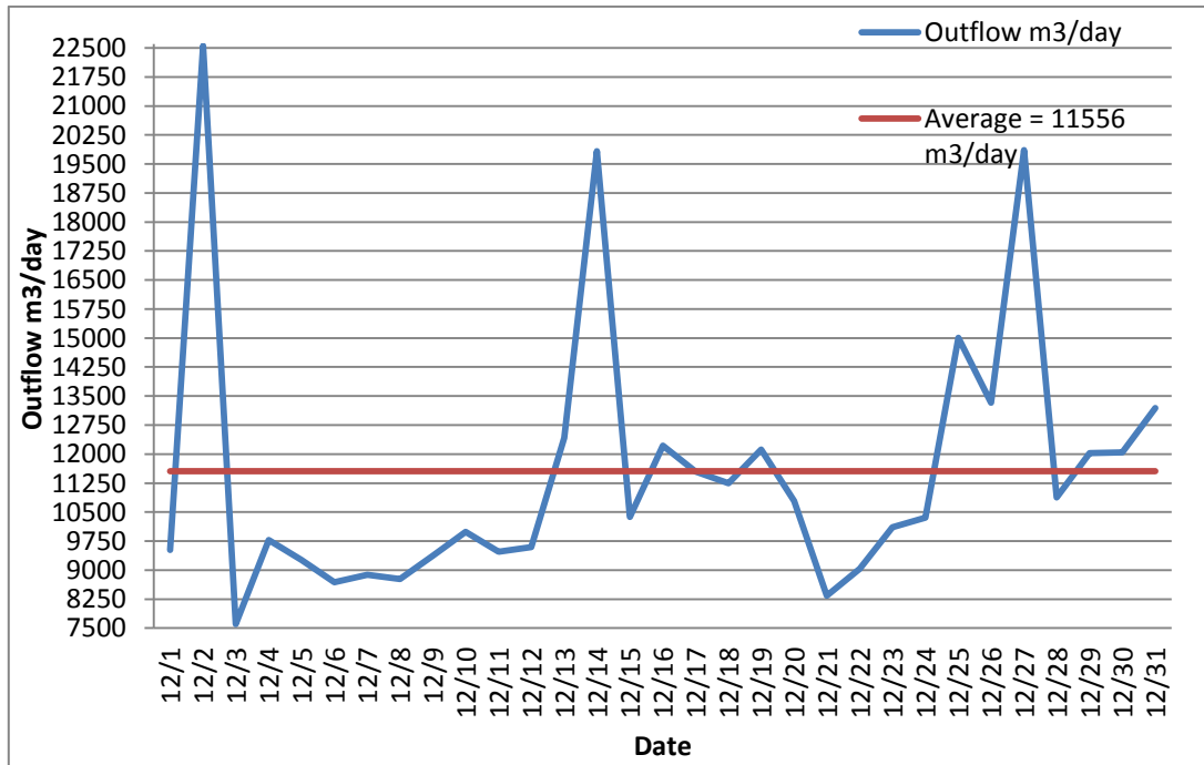
شكل (3) : كمية المياه المعالجة الخارجة من المحطة
