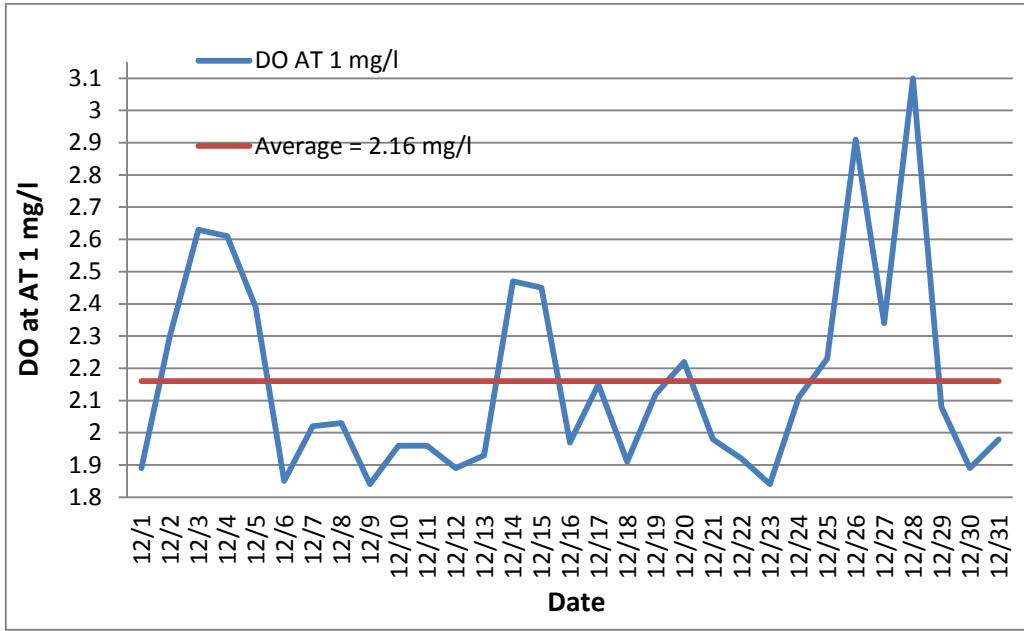
شكل (4) : كمية الأوكسجين المذاب في خزان التهويه 240.1
