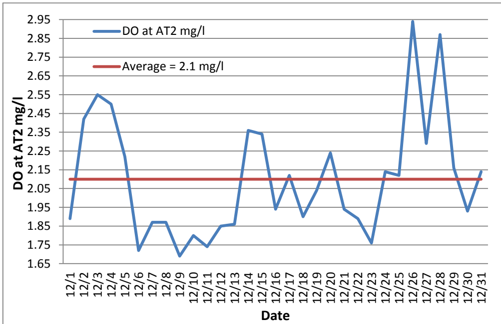
شكل (5) : كمية الأوكسجين المذاب في خزان التهويه 240.2
