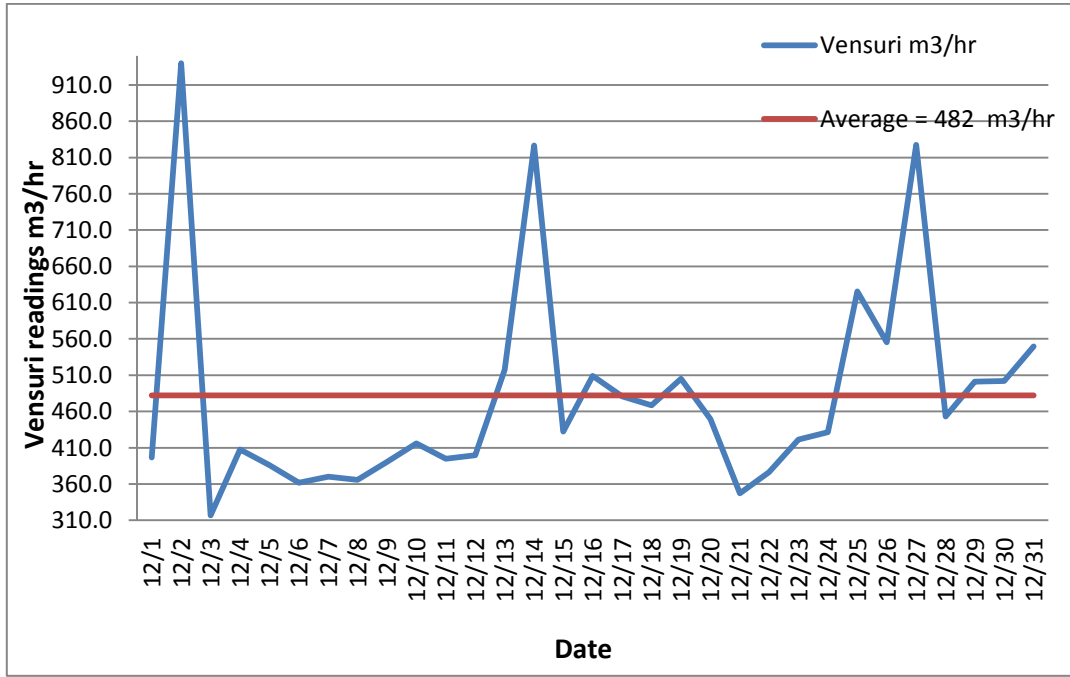
شكل (2) : معدل قراءة عداد فنتشوري (Venture)
