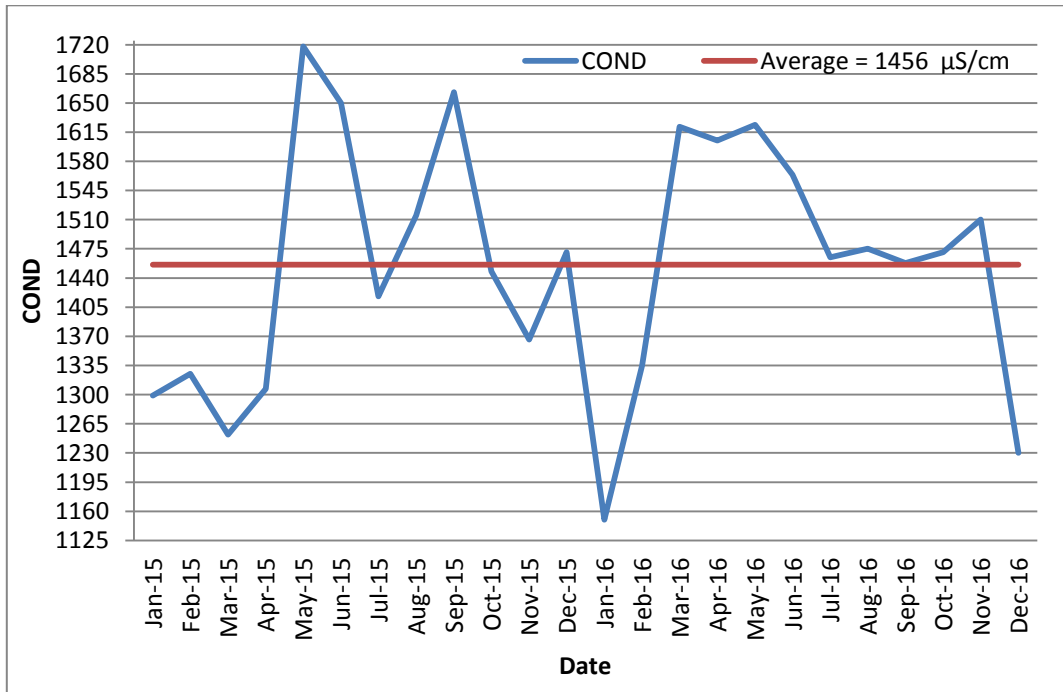
الشكل (15) : معدل قيم التوصيلية الكهربائية الشهرية للمياه العادمة الداخلة لمحطة المعالجة
