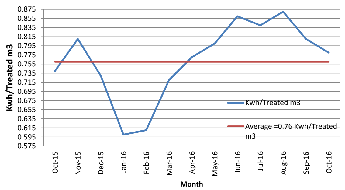
الشكل (18) : كميات الطاقة الكهربائية المستخدمة بدلالة كيلو واط ساعة لكل متر مكعب مياه معالجة
