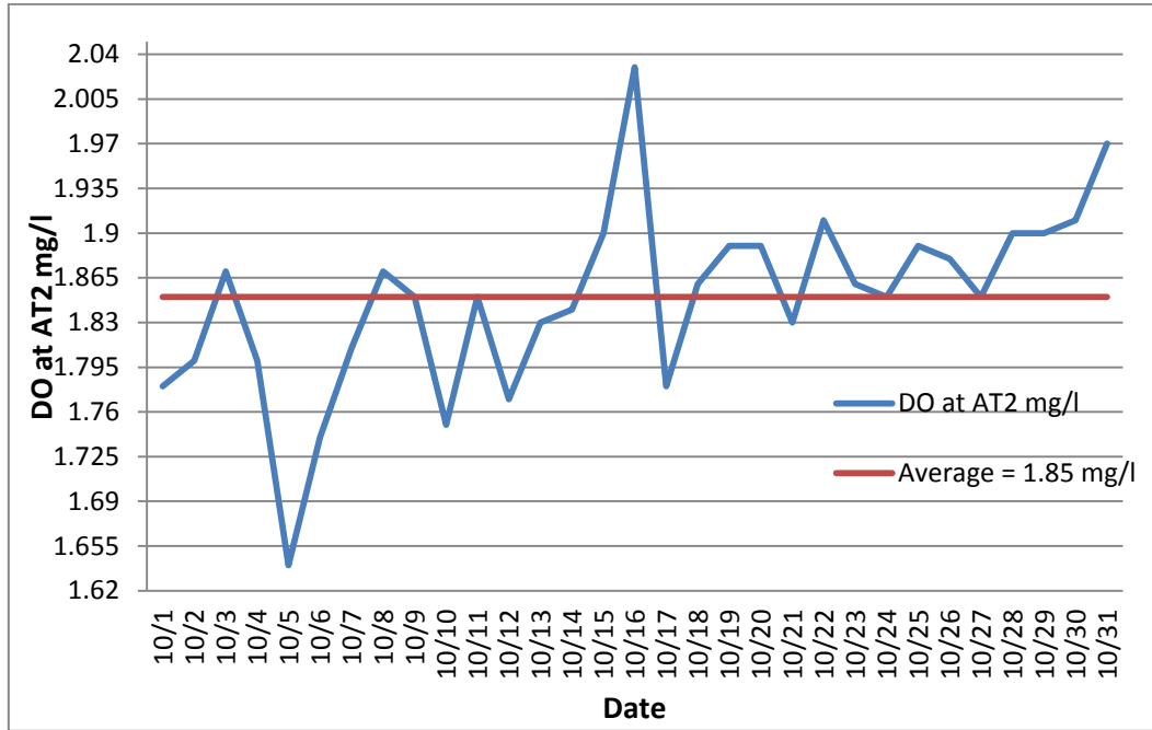
شكل (4) : كمية الأكسجين المذاب في خزان التهويه 240.1
