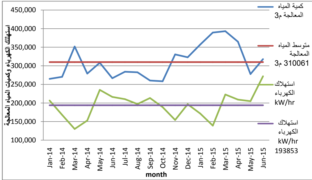
الشكل (14) : معدلي استهلاك الكهرباء والمياه المعالجة
