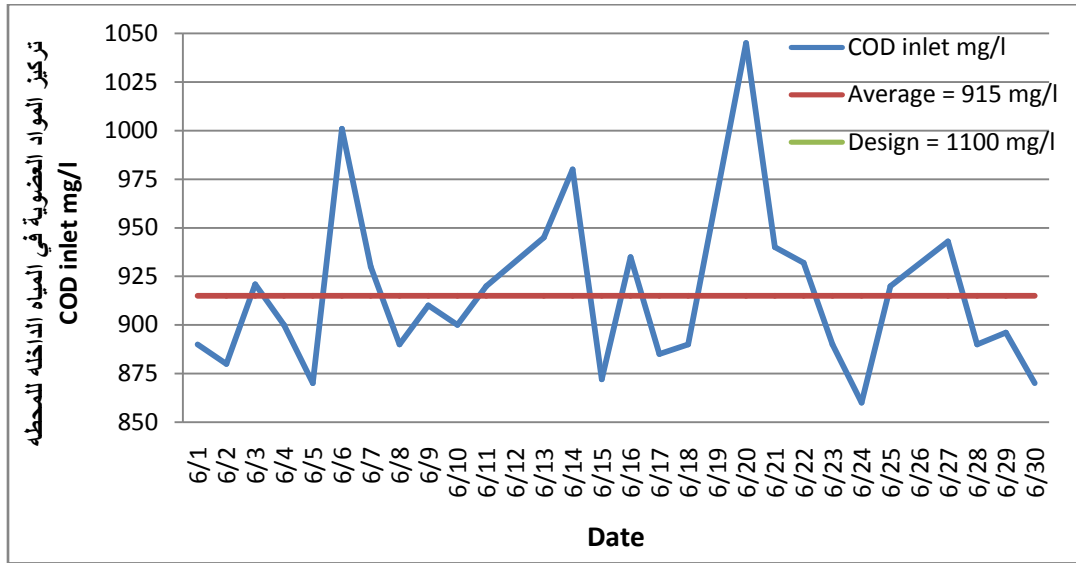
شكل (6) : تركيز المواد العضوية في المياه العادمة الداخلة للمحطة
