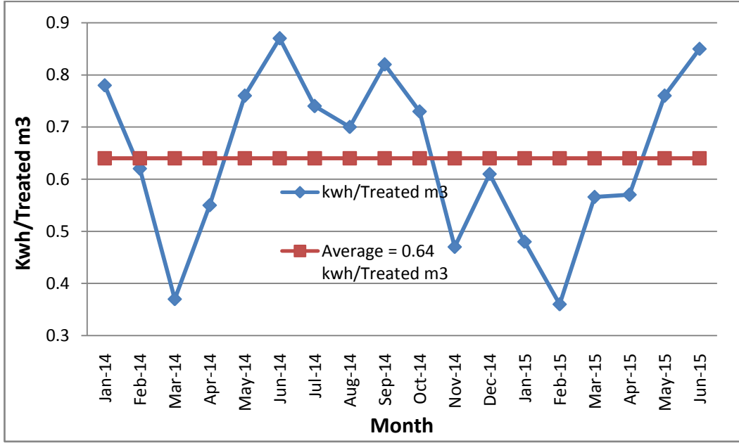
الشكل (19) : كميات الطاقة الكهربائية المستخدمة بدلالة كيلو واط ساعة لكل متر مكعب مياه معالجة
