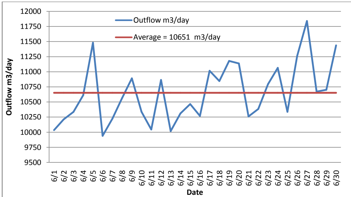
شكل (3) : كمية المياه العادمة الخارجة من المحطة
